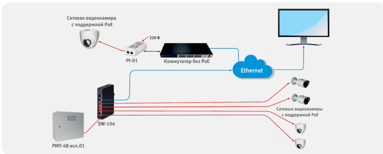
Рисунок 71. Организация электропитания сетевой системы видеонаблюдения с использованием технологии PoE
