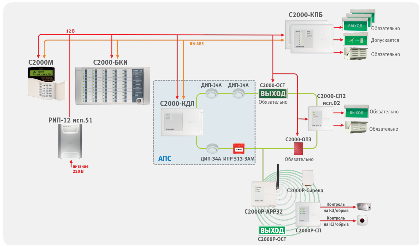
Рисунок 15. Пример СОУЭ 1-го и 2-го типов на базе блочно-модульного ППКУП с адресно-аналоговой СПС
