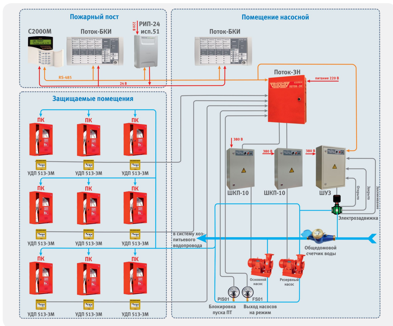
Рисунок 23. Внутренний противопожарный водопровод
