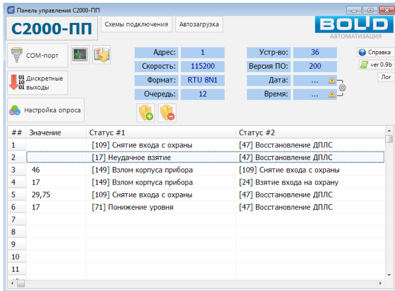
Рисунок 81. Панель управления «С2000-ПП»
