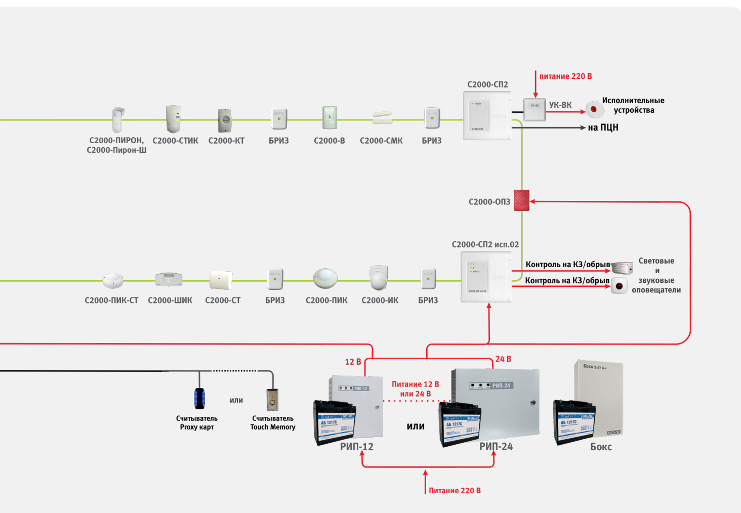
Рисунок 36. Адресная система охранной сигнализации
