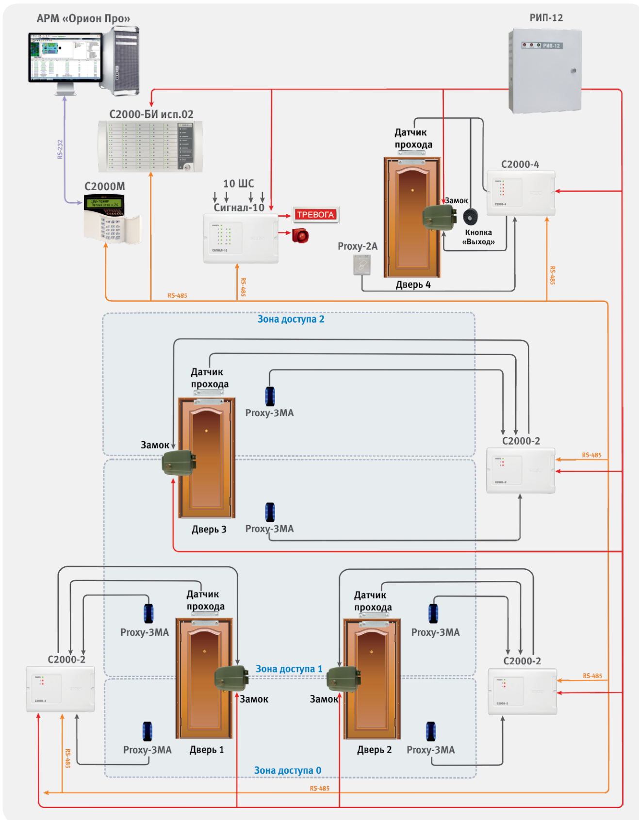
Рисунок 50. Сетевая СКУД с использованием программного обеспечения
