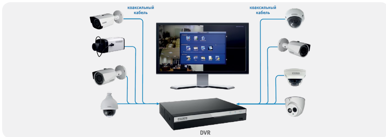
Рисунок 54. Аналоговое видеонаблюдение с локальным рабочим местом
