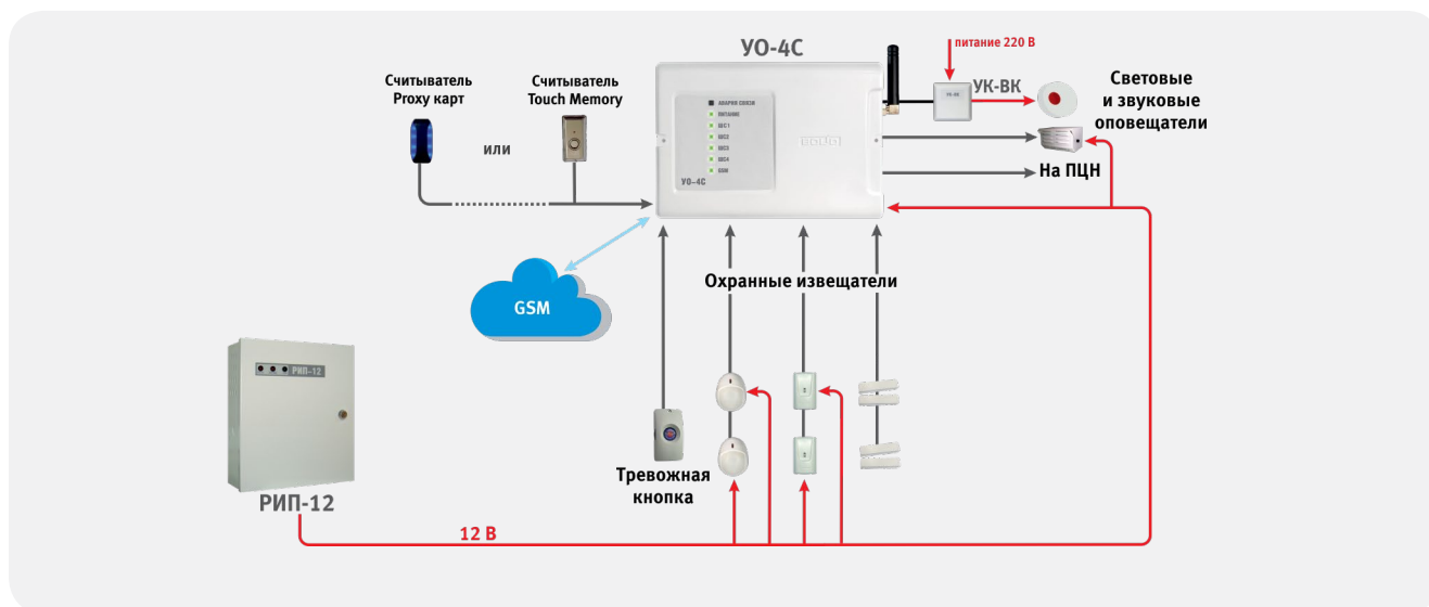
Рисунок 33. Автономное использование «УО-4С»
