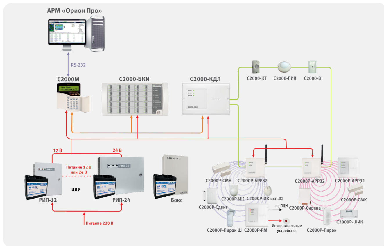
Рисунок 37. Адресная радиоканальная система на основе «С2000Р-APP32»
