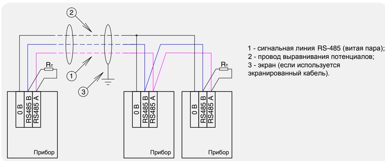
Рисунок 95. Схема подключения приборов к магистральному интерфейсу RS-485
