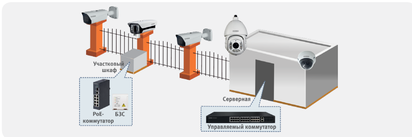
Рисунок 72. Типовые подходы к проектированию охраны протяженных периметров
