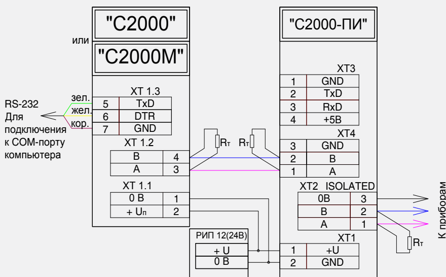
Рисунок 85. Схема подключения пультов «С2000»/ «С2000М» к персональному компьютеру с АРМ «Орион Про» с гальванической изоляцией интерфейса RS-485
