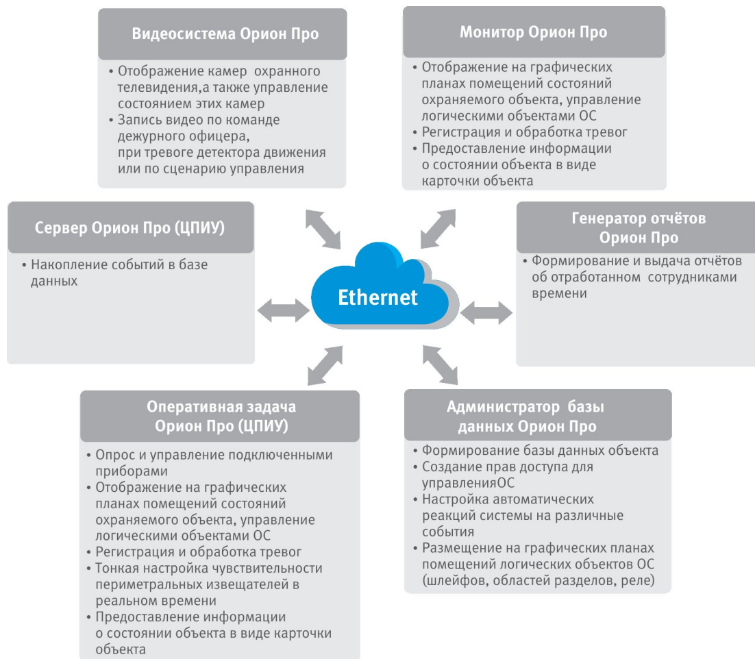
Рисунок 40. Функционал модулей программного обеспечения
