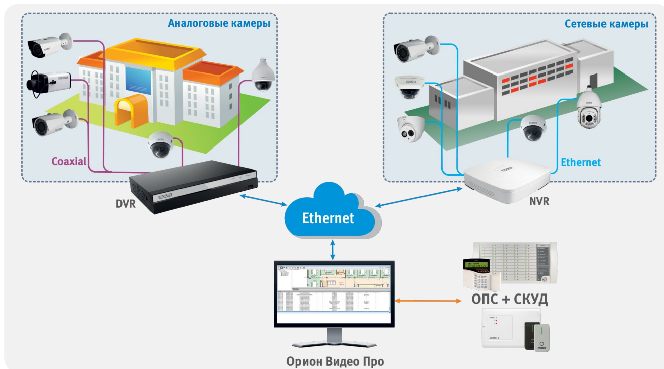
Рисунок 57. Аналоговое и/или сетевое видеонаблюдение с удаленным рабочим местом на АРМ «Орион Про»
