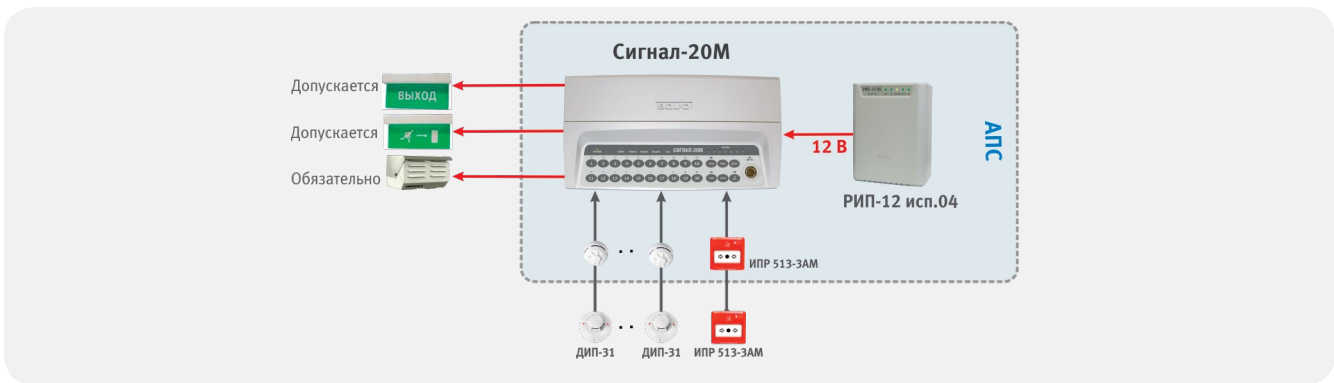
Рисунок 14. Пример СОУЭ 1-го типа на базе прибора «Сигнал-20М»
