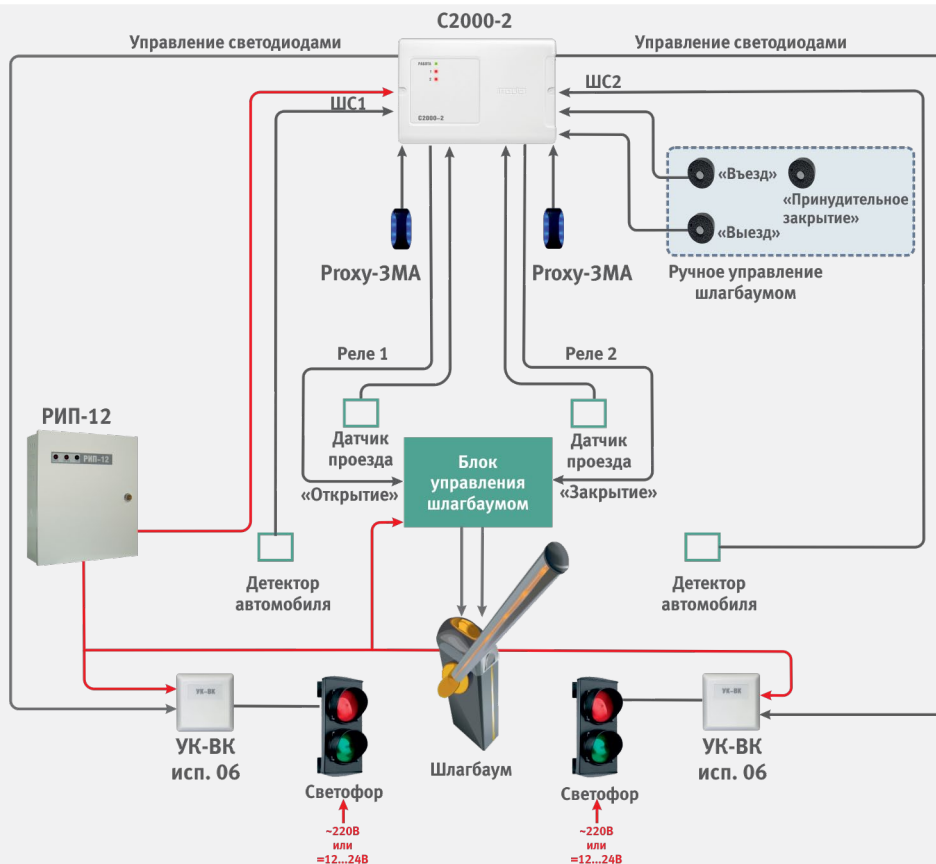
Рисунок 44. Режим работы «Шлагбаум»
