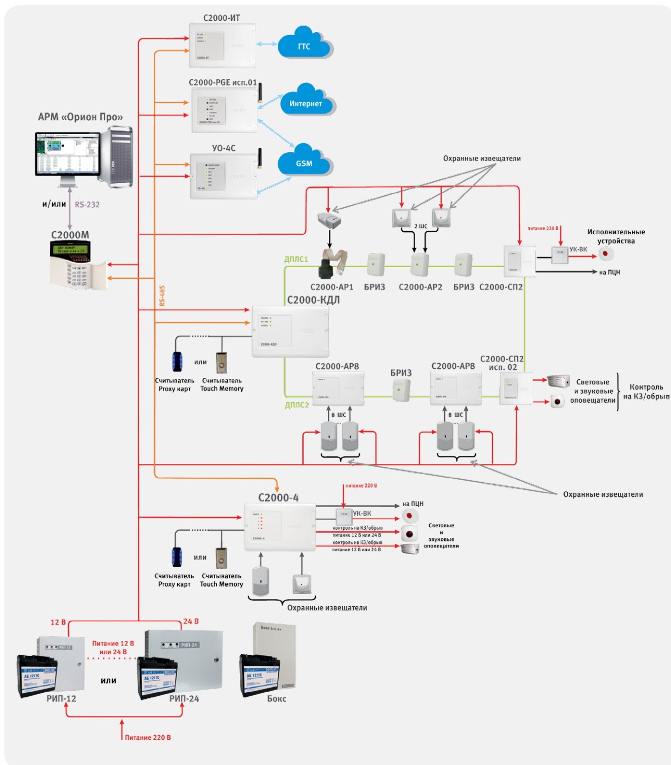
Рисунок 38. Комбинированная система охранной сигнализации
