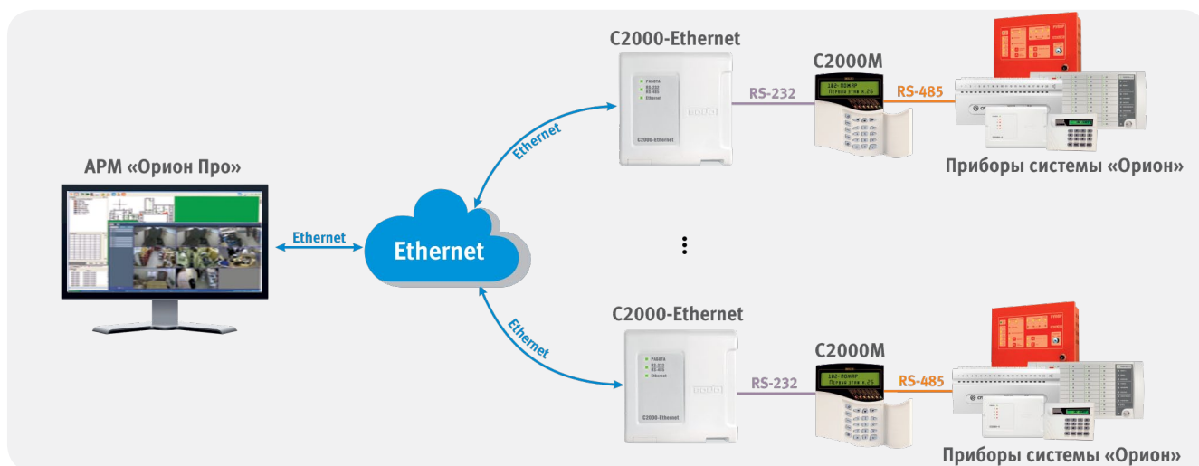
Рисунок 88. Типовая схема работы «C2000-Ethernet» по протоколу «Орион Про»
