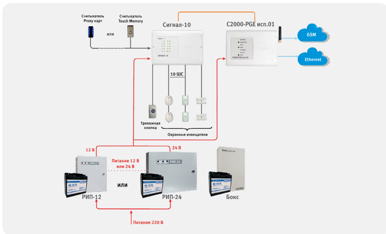
Рисунок 34. Система охранной сигнализации на базе прибора «Сигнал-10» и устройства «С2000-PGE исп.01»
