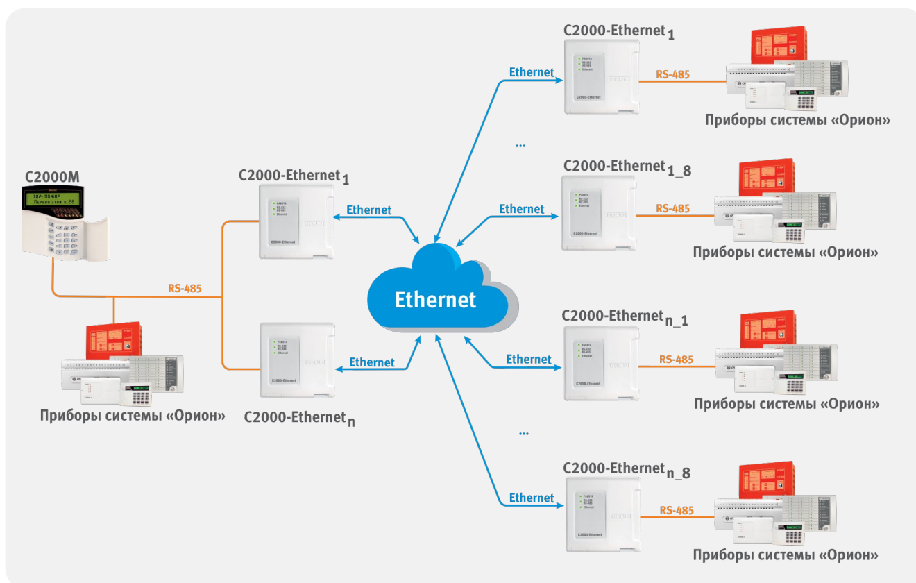
Рисунок 99. Структурная схема использования «C2000-Ethernet» с «C2000M»
