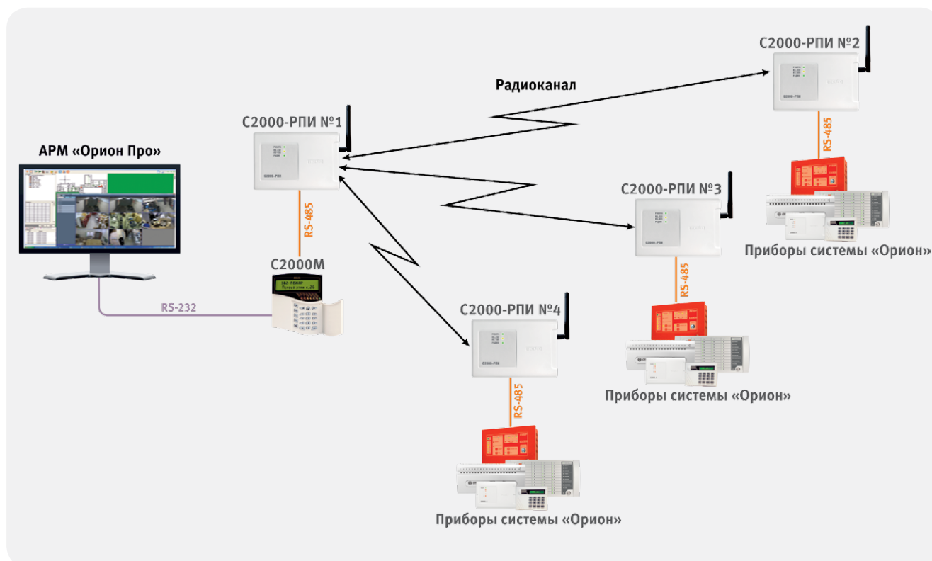
Рисунок 102. Структурная схема использования «С2000-РПИ» с АРМ «Орион Про» и «С2000М», соединение «точка-многоточка»
