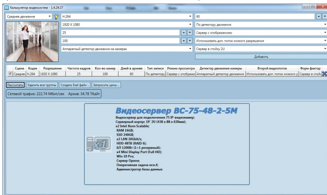
Рисунок 67. Пример рабочего интерфейса утилиты «Калькулятор видеосистемы» производства компании БОЛИД
