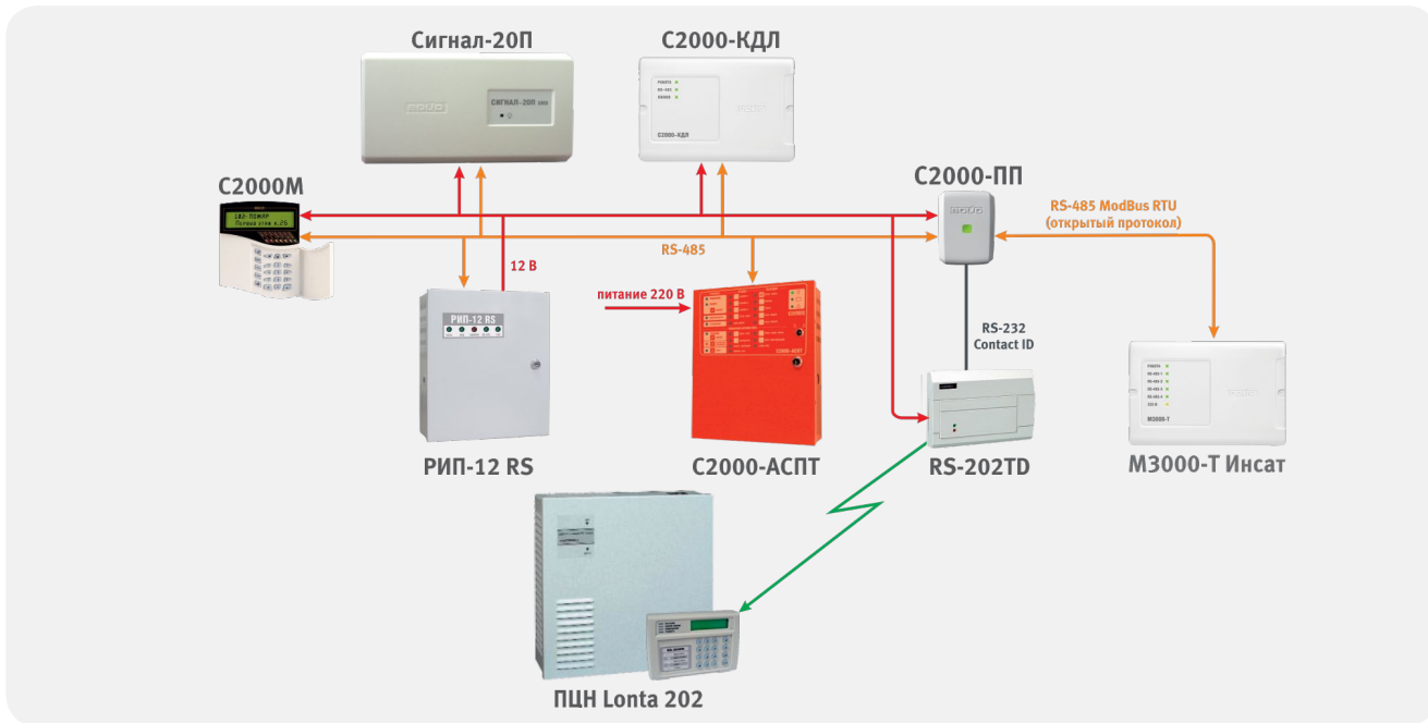
Рисунок 79. Применение «С2000-ПП» в ведомом режиме
