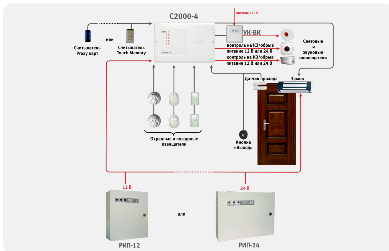
Рисунок 47. «С2000-4» с функционалом контроля доступа
