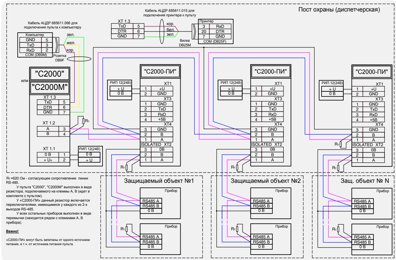
Рисунок 98. Построение сети RS-485 с топологией «звезда» при помощи повторителей
