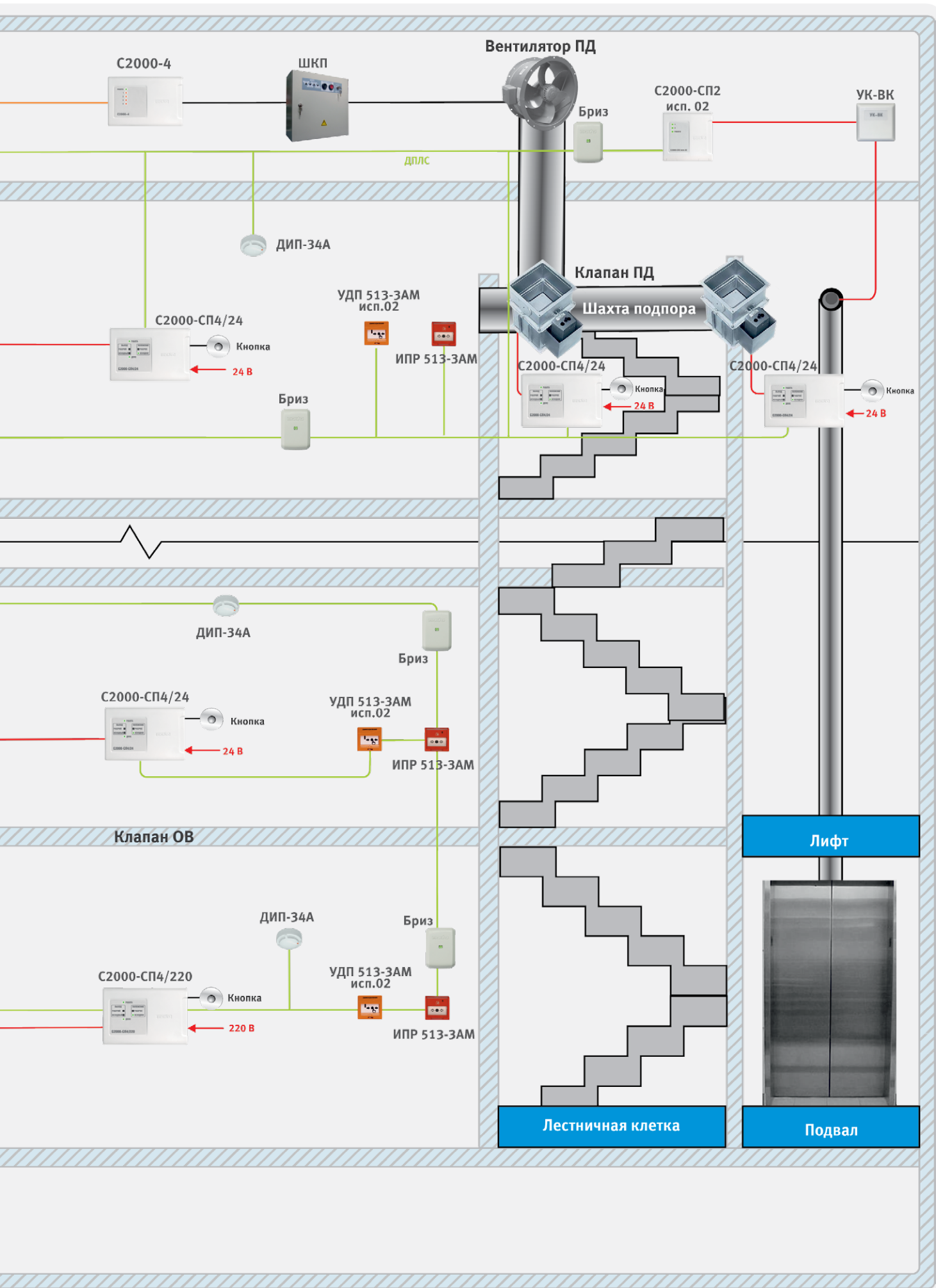
Рисунок 27. Структурная схема управления противопожарными клапанами
