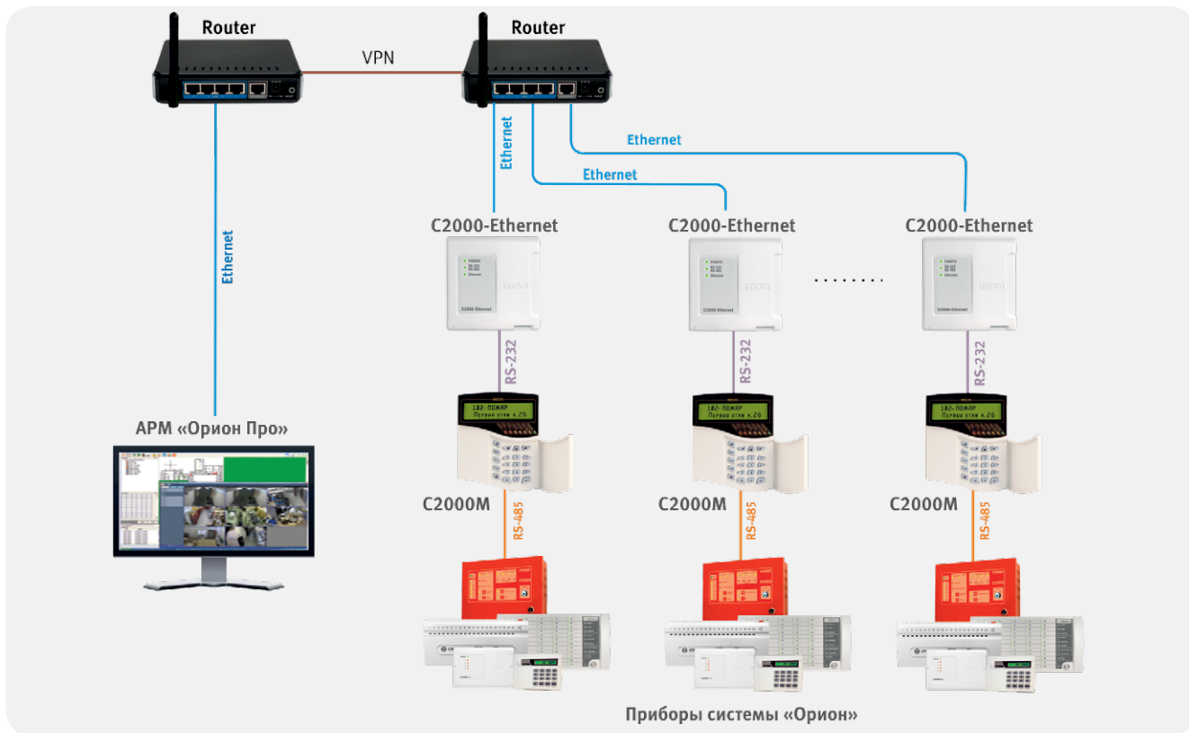
Рисунок 89. Пример использования «C2000-Ethernet» в глобальных сетях
