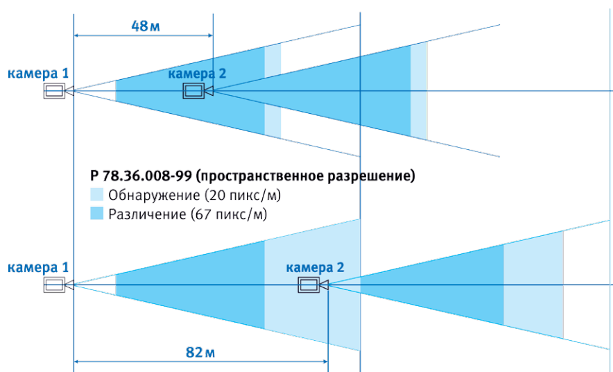
Рисунок 73. Варианты перекрытий зон обзора на протяженном периметре
