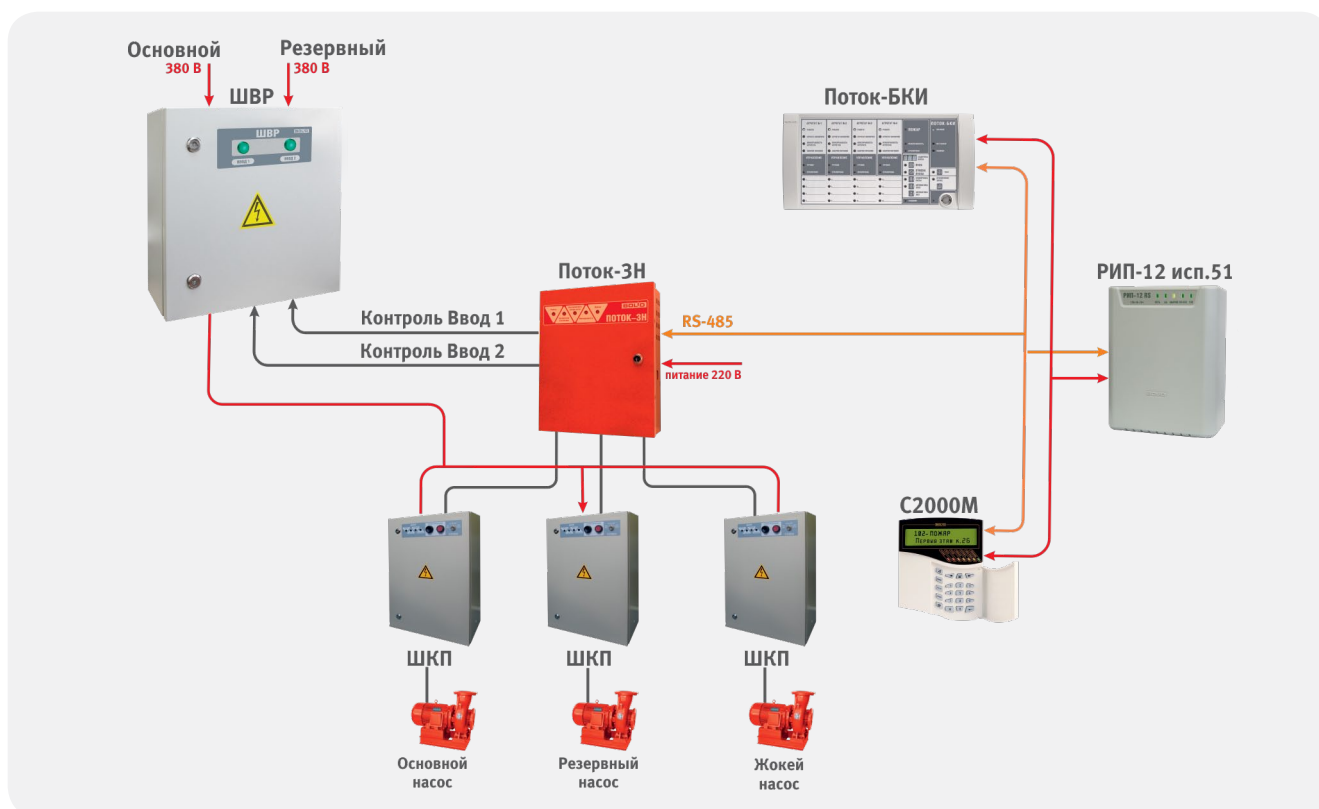
Рисунок 29. ШВР в составе ППУ
