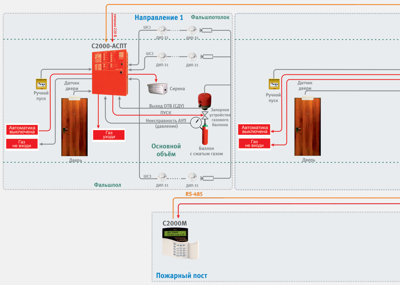
Рисунок 20. Распределенная установка газового пожаротушения
