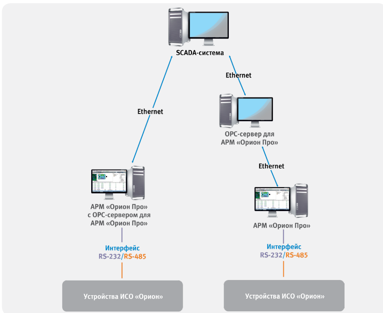
Рисунок 83. Передача данных в SCADA-систему
