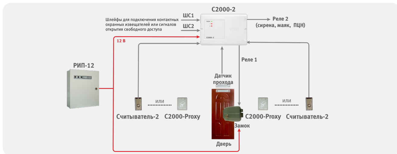
Рисунок 42. Режим работы «Одна дверь на вход/выход»
