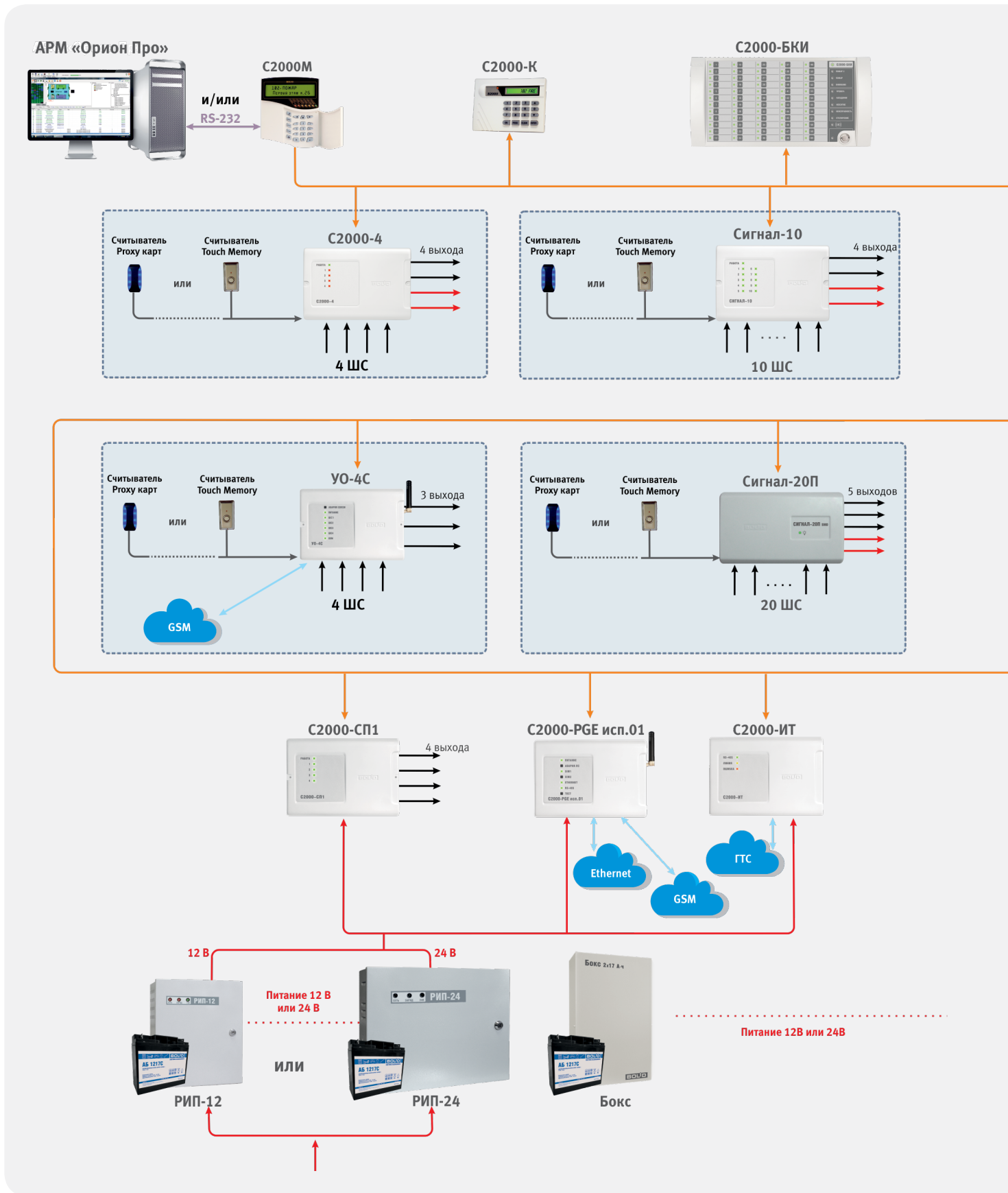
Рисунок 35. Система охранной сигнализации с сетевым контроллером
