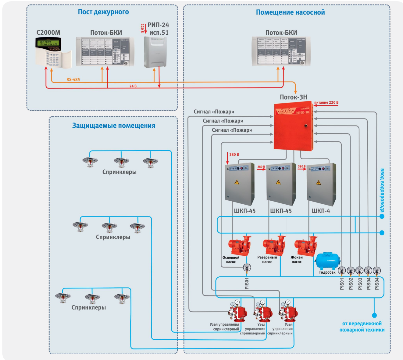
Рисунок 24. Автоматическая установка пожаротушения с тремя спринклерными секциями
