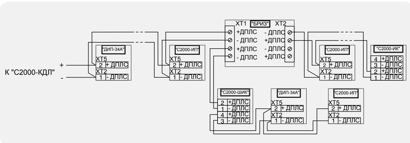
Рисунок 109. Схема подключения адресных устройств в ДПЛС с топологией построения «дерево»
