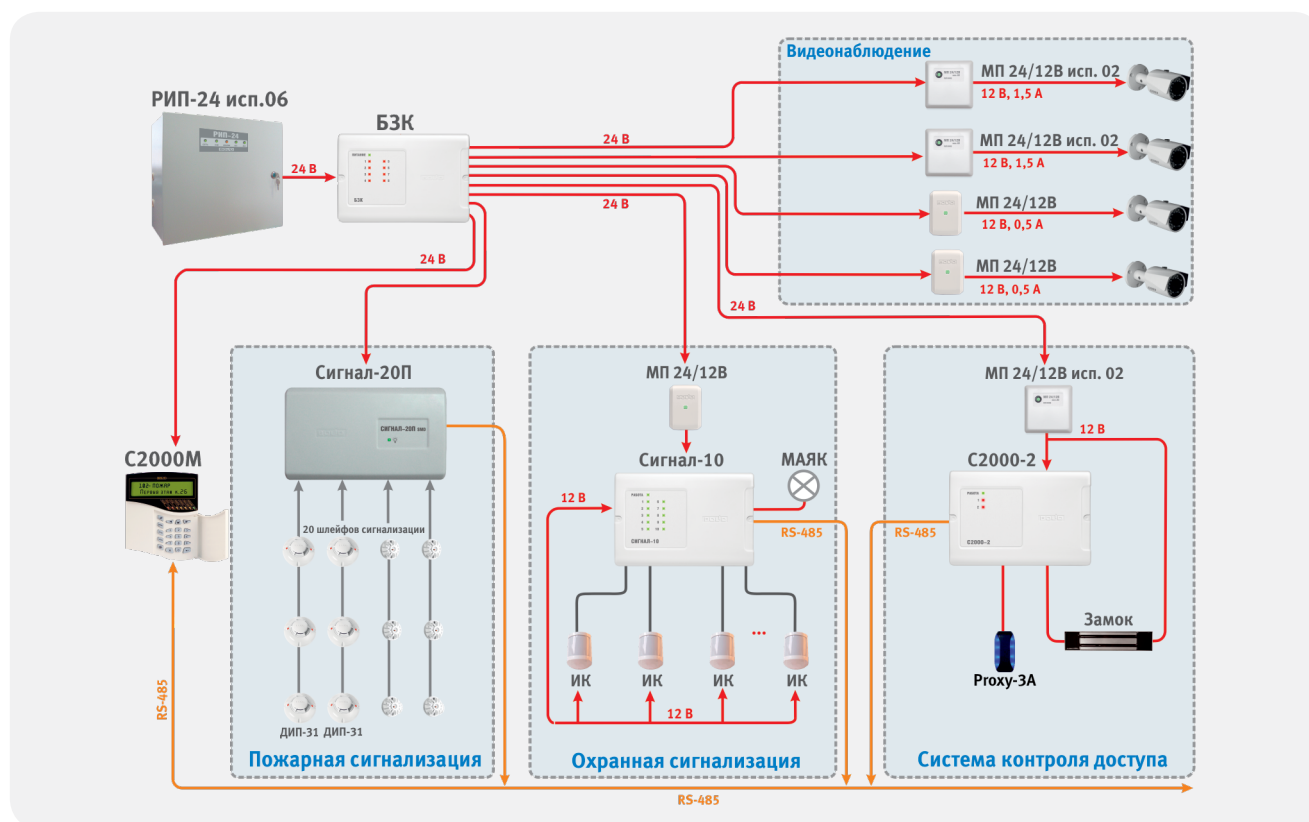
Рисунок 77. Организация электропитания интегрированных систем
