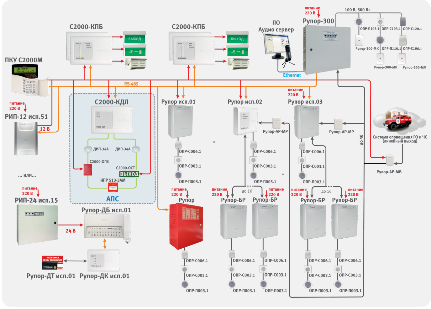
Рисунок 17. Пример СОУЭ 4-го типа с автономным комплексом обратной связи
