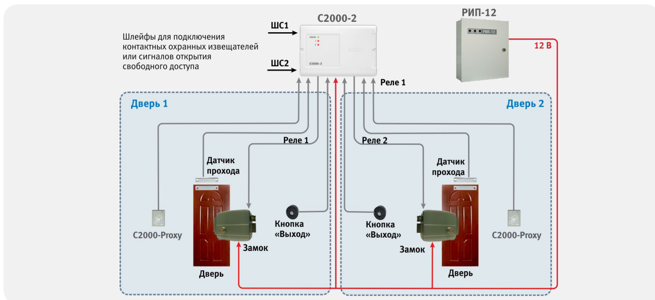
Рисунок 41. Режим работы «Две двери на вход»
