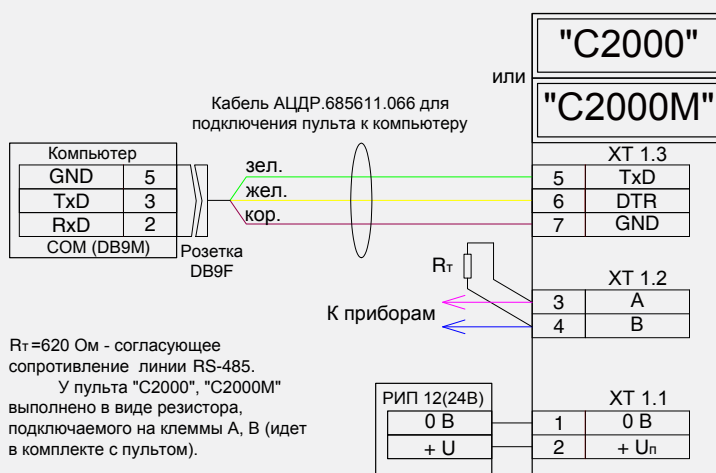
Рисунок 84. Схема подключения пульта «С2000»/ «С2000М» к персональному компьютеру с АРМ «Орион Про»
