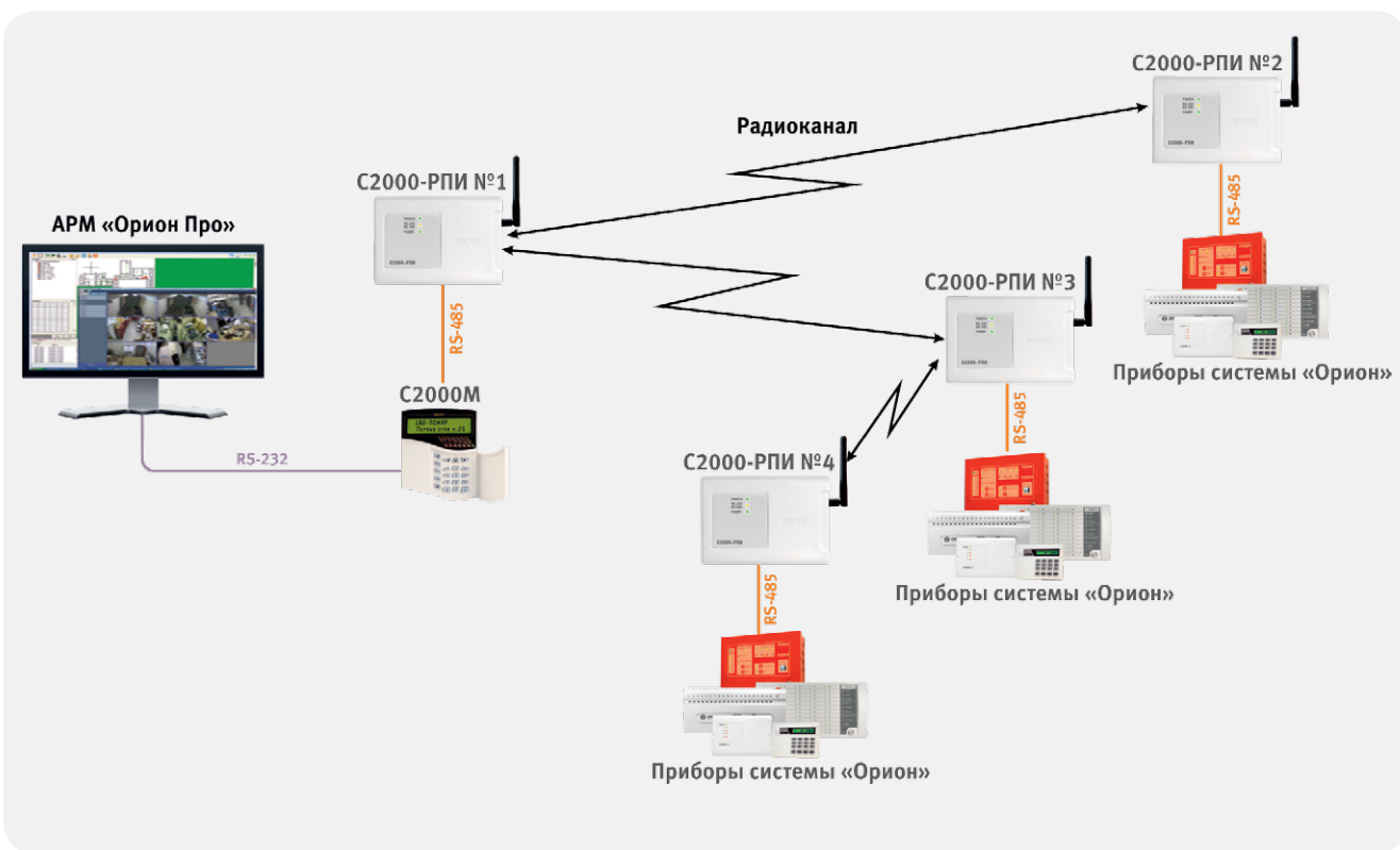
Рисунок 103. Структурная схема использования «С2000-РПИ» с АРМ «Орион Про» и «С2000М», соединение «точка-многоточка» с ретрансляцией
