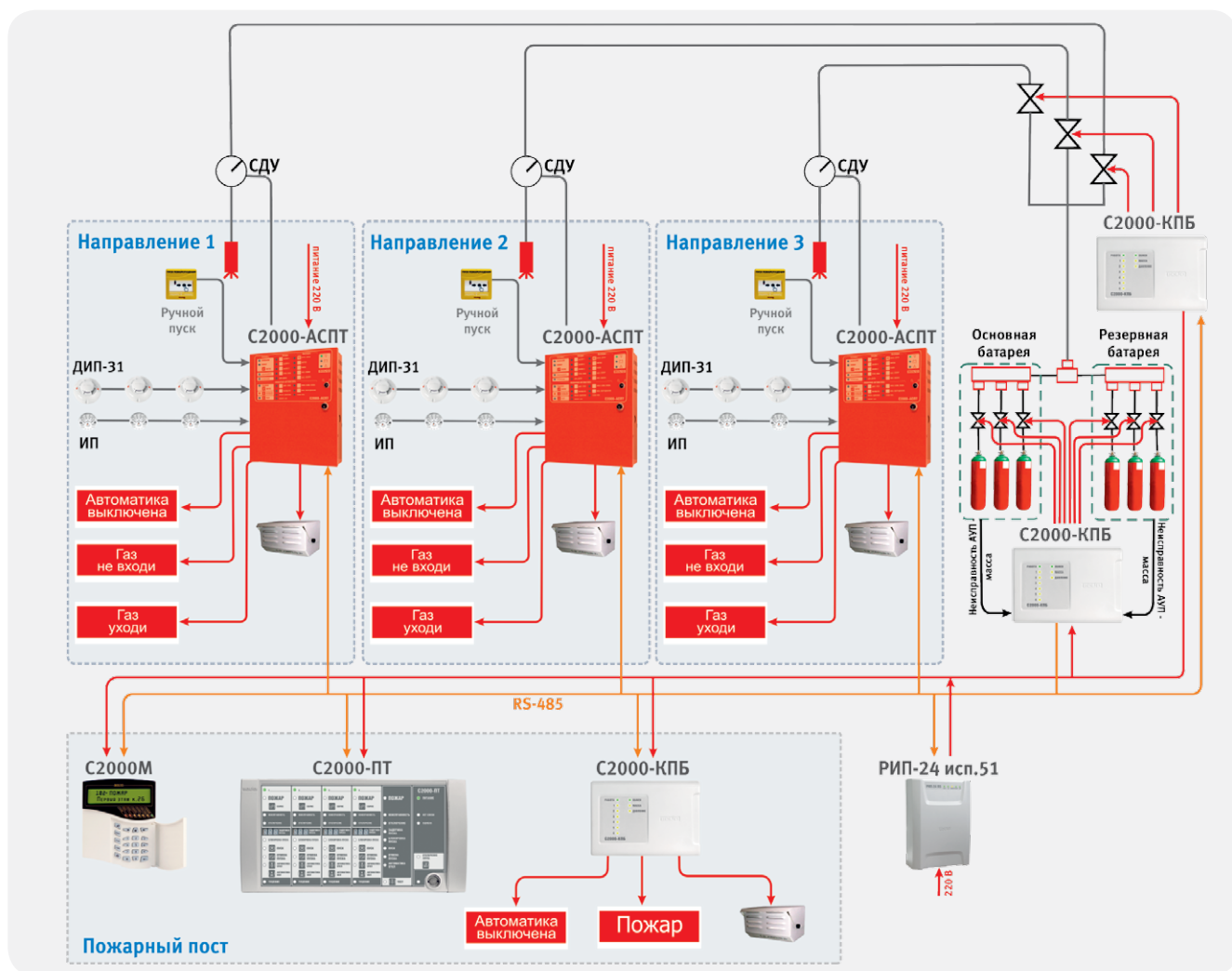
Рисунок 21. Централизованная система автоматического пожаротушения с газовой батареей при использовании электромеханических запорных клапанов
