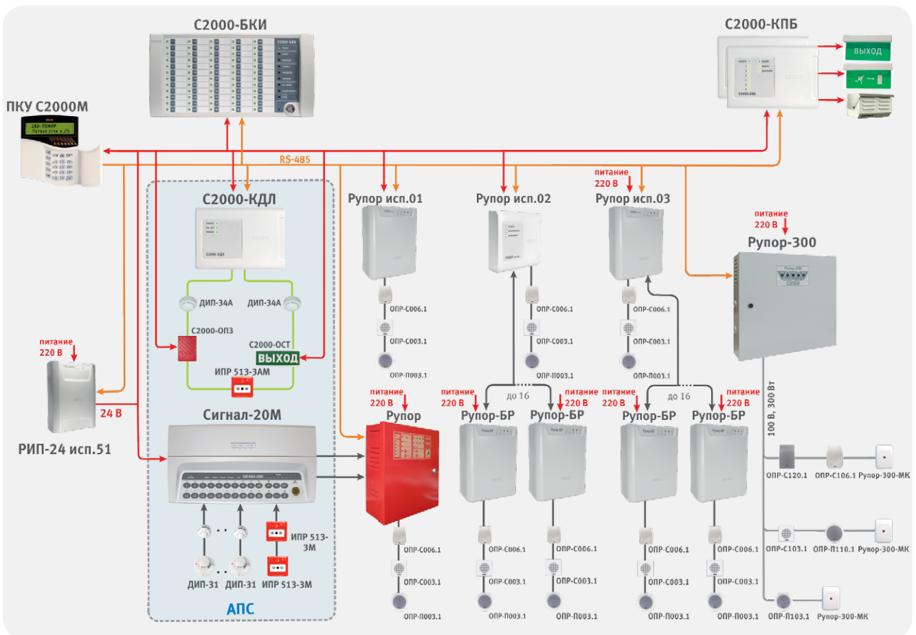
Рисунок 16. Пример СОУЭ 3-го типа с несколькими зонами оповещения
