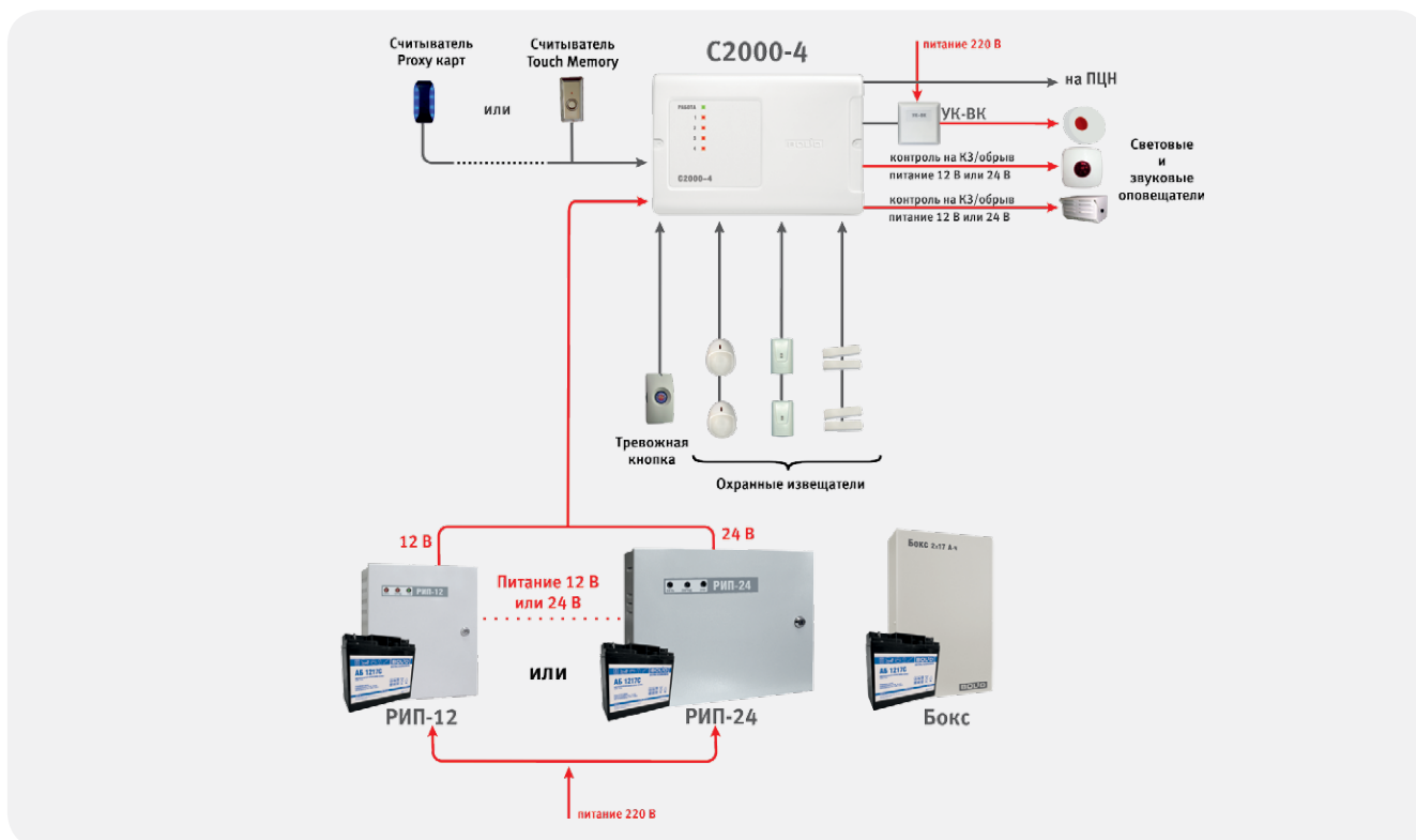
Рисунок 30. Автономное использование блока «С2000-4»
