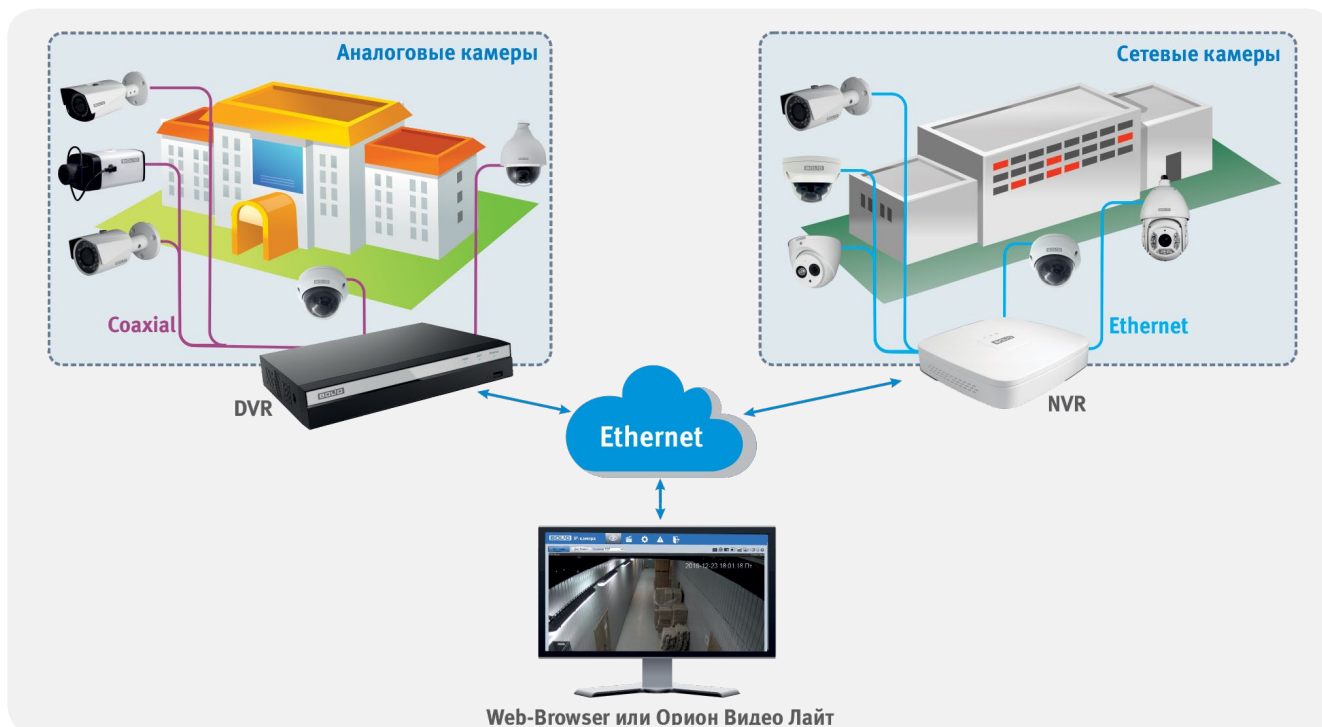
Рисунок 56. Аналоговое и/или сетевое видеонаблюдение с удаленным рабочим местом через программу Web-Browser или Орион Видео Лайт
