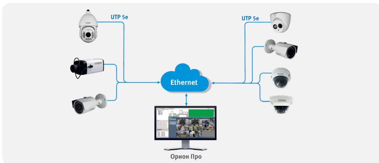
Рисунок 58. Сетевое видеонаблюдение напрямую с сетевых камер с удаленным рабочим местом на АРМ «Орион Про»
