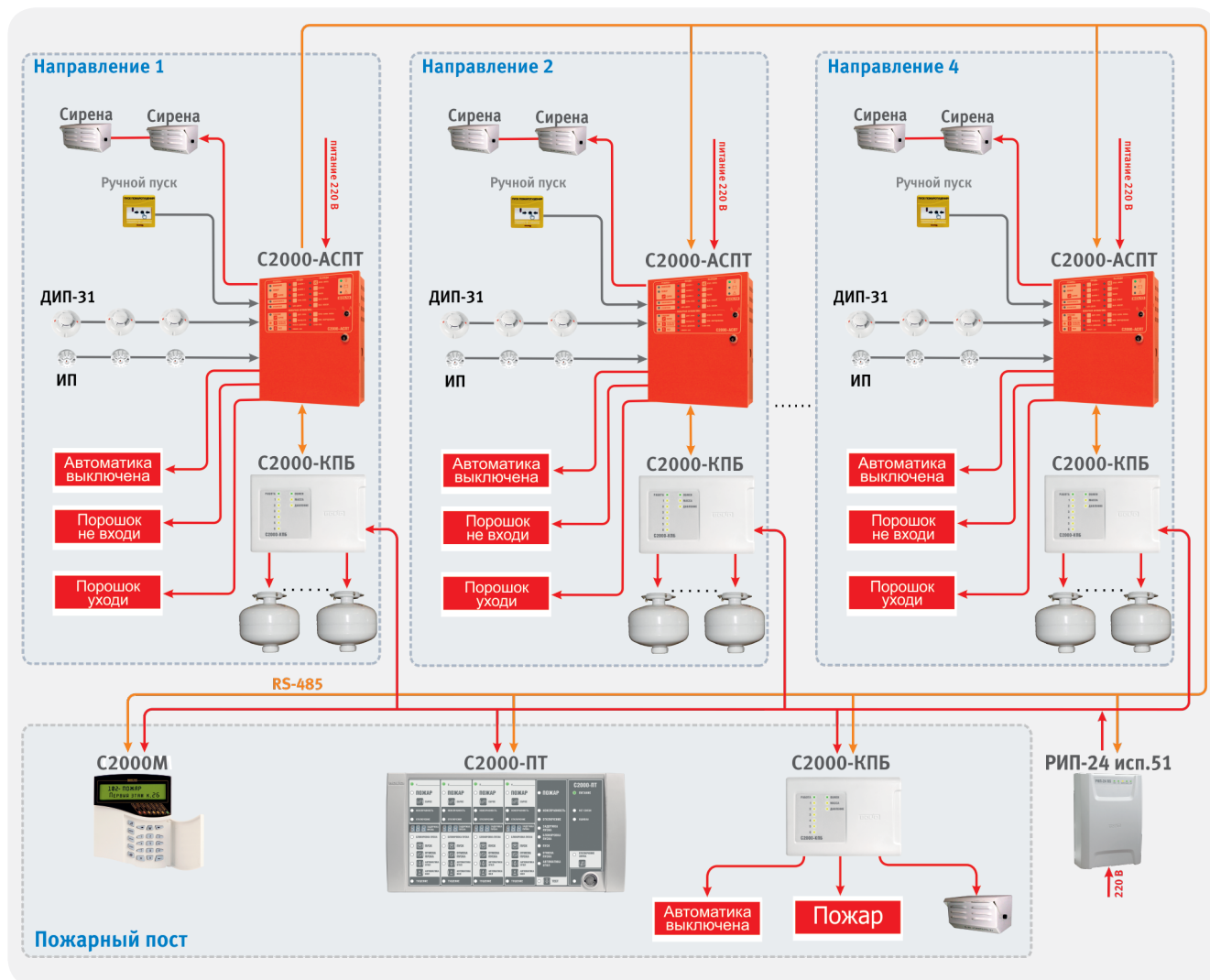
Рисунок 22. Система порошкового пожаротушения
