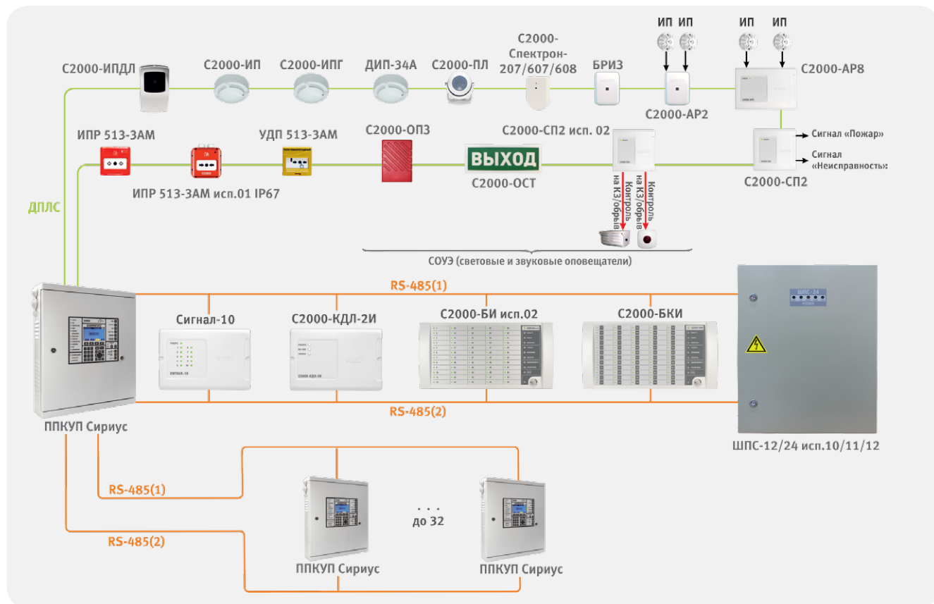
Рисунок 10. Система АПС с повышенными требованиями к надежности
