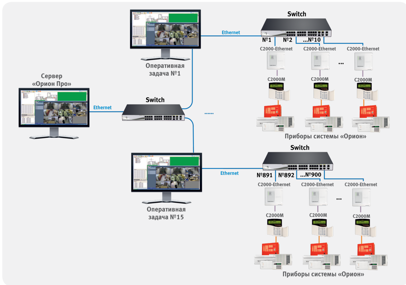
Рисунок 90. Пример построения системы с использованием «C2000-Ethernet» на 900 объектах
