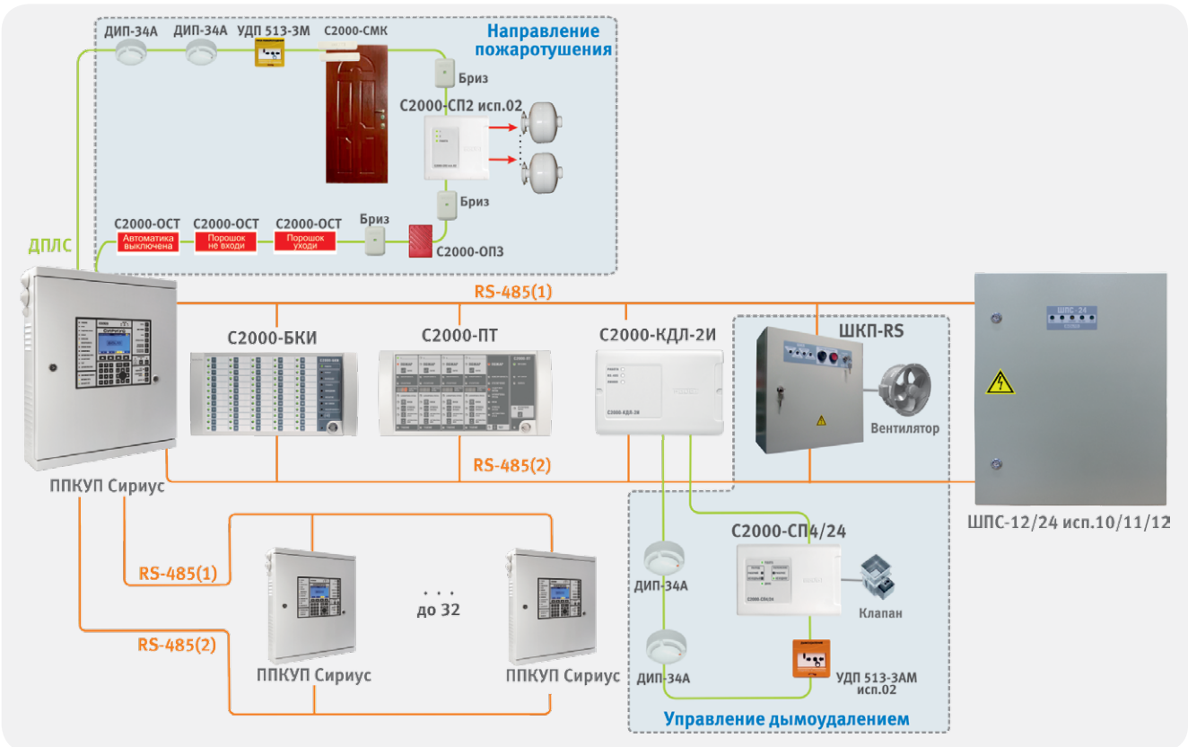
Рисунок 28. Система управление пожаротушением и дымоудалением с повышенным требованиями к надежности
