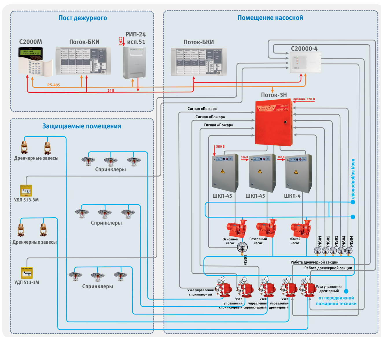
Рисунок 25. Автоматическая установка пожаротушения с тремя спринклерными и двумя дренчерными секциями
