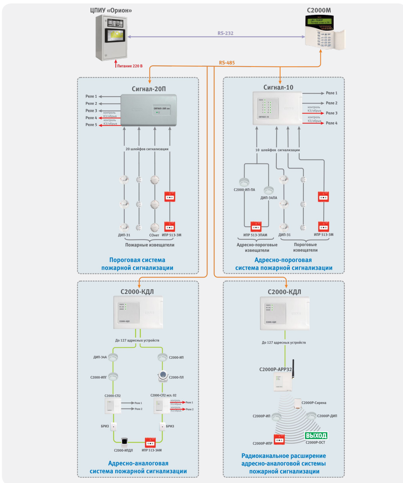
Рисунок 2. Типы систем пожарной сигнализации
