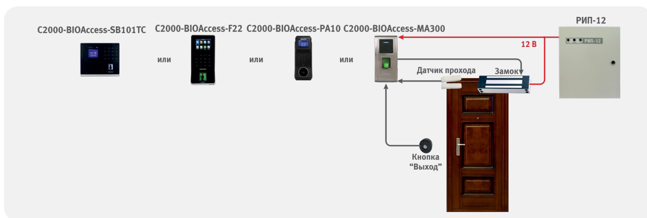
Рисунок 48. Биометрическая СКУД
