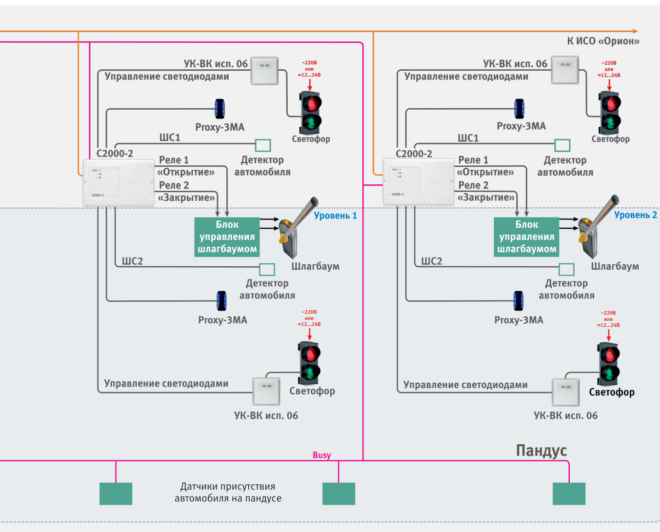
Рисунок 46. Организация въезда на двухуровневую парковку
