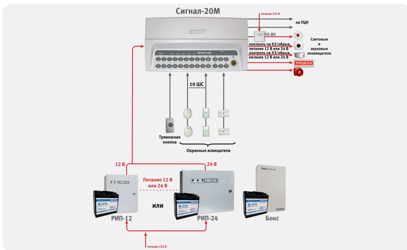
Рисунок 32. Автономное использование прибора «Сигнал-20М»
