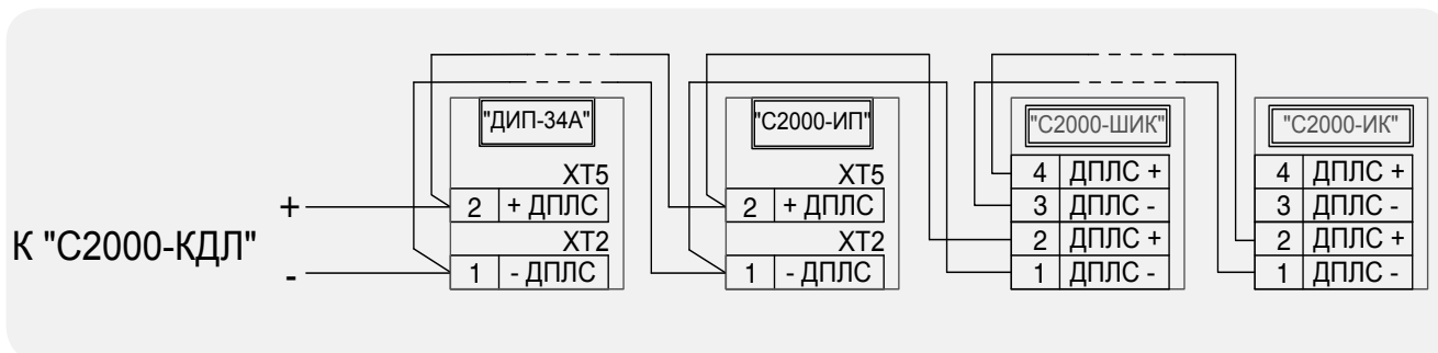
Рисунок 108. Схема подключения адресных извещателей в ДПЛС с топологией построения «шина»
