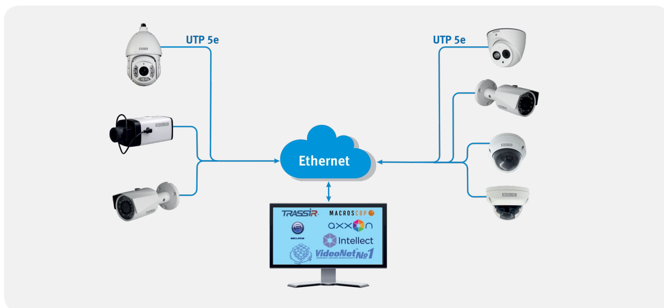
Рисунок 59. Сетевое видеонаблюдение напрямую с сетевых камер с удаленным рабочим местом на сторонних системах видеорегистрации
