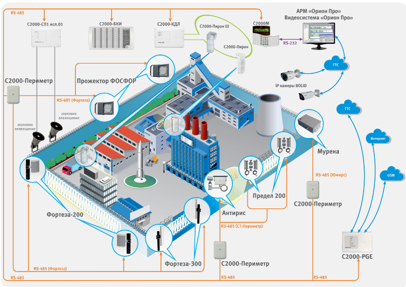
Рисунок 39. Система охраны периметра
