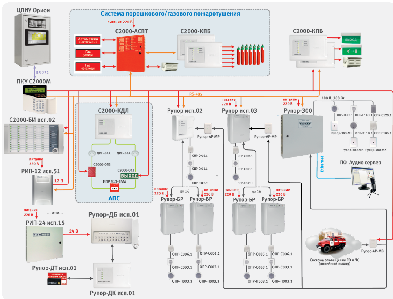
Рисунок 18. СОУЭ 5-го типа с комплексом обратной связи, входящим в состав ИСО «Орион»
