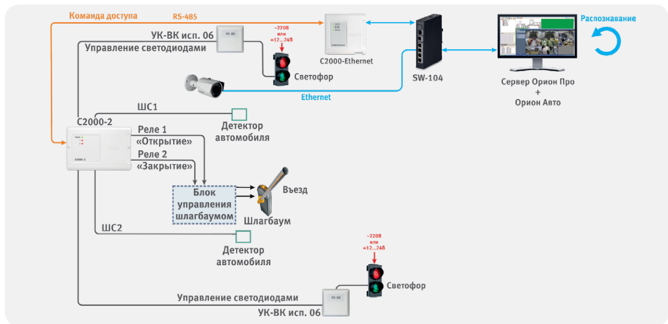
Рисунок 74. Видеонаблюдение с определением номеров на транспортном КПП
