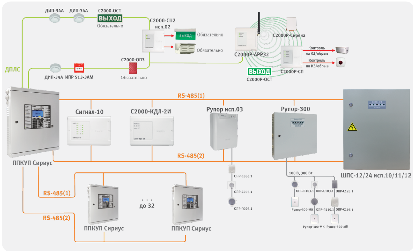
Рисунок 19. Система оповещения с повышенными требованиями к надежности
