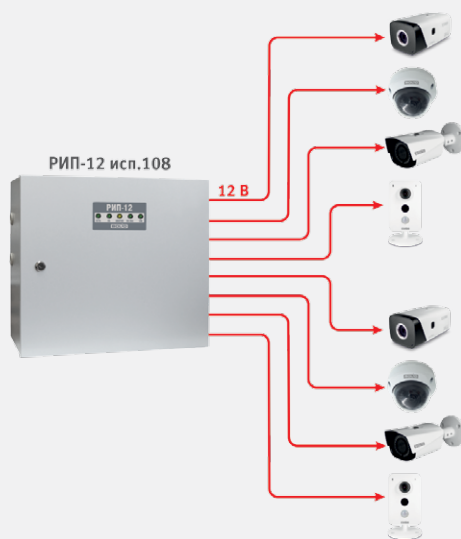
Рисунок 69. Организация питания видеокamер с помощью многоканального источника резервированного питания РИП-12 исп.108
