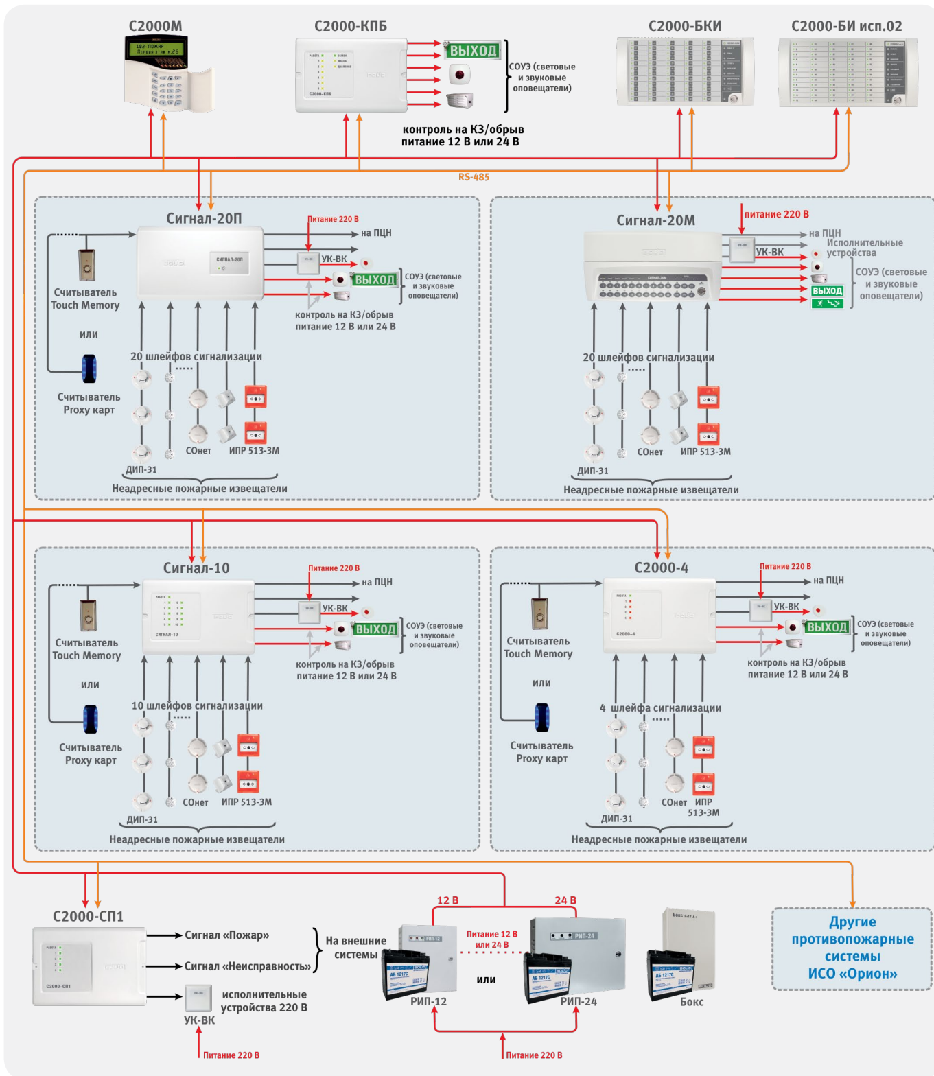
Рисунок 4. Неадресная система пожарной сигнализации в ИСО «Орион»
