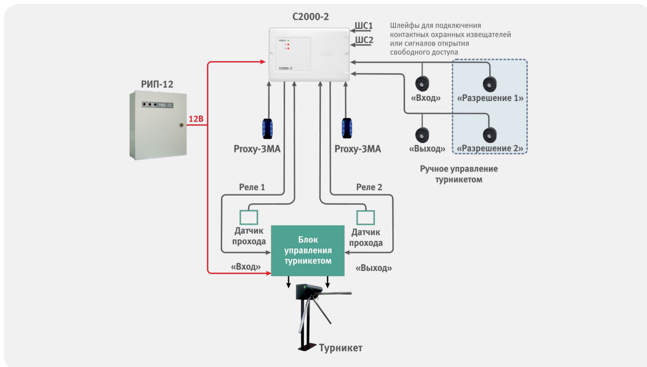
Рисунок 43. Режим работы «Турникет»
