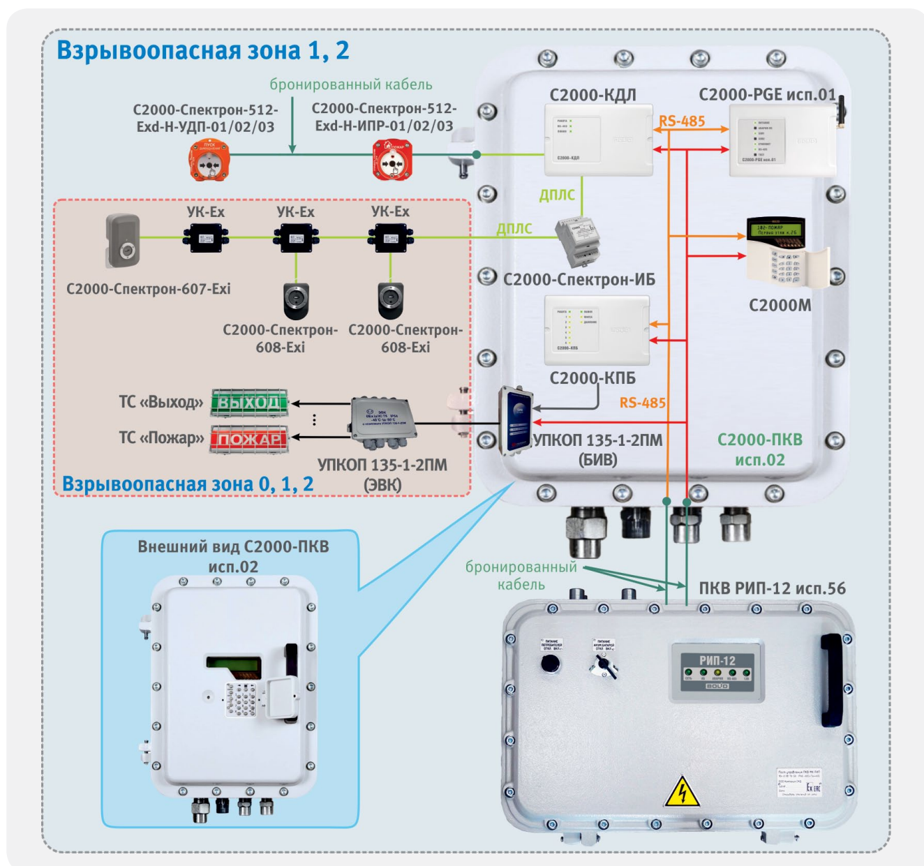
Рисунок 9. Размещение оборудования АПС внутри взрывоопасной зоны
