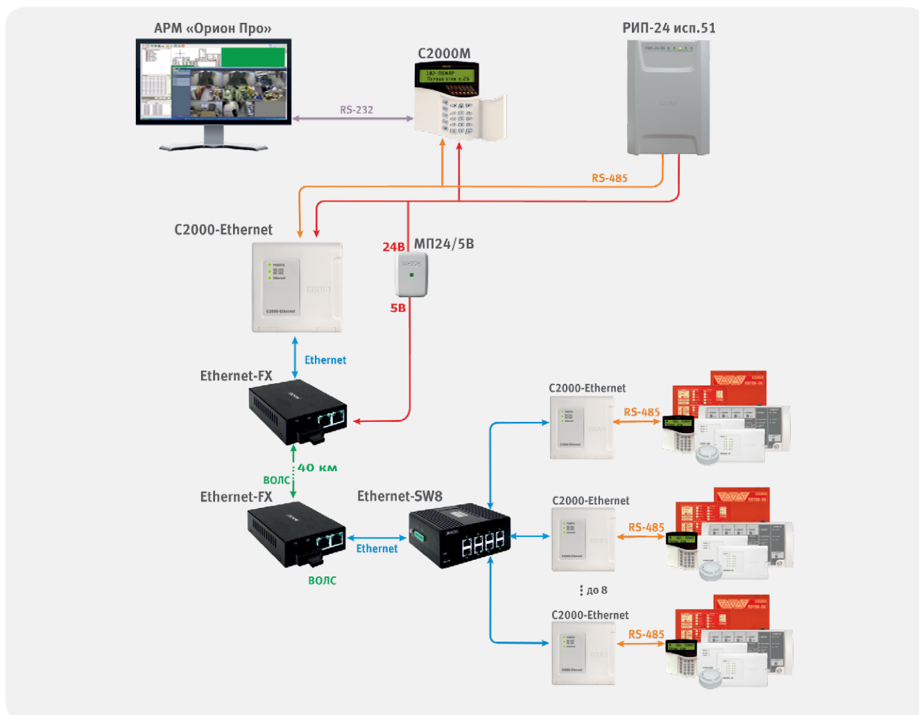
Рисунок 111. Каналообразующее оборудование для систем пожарной сигнализации и автоматики
