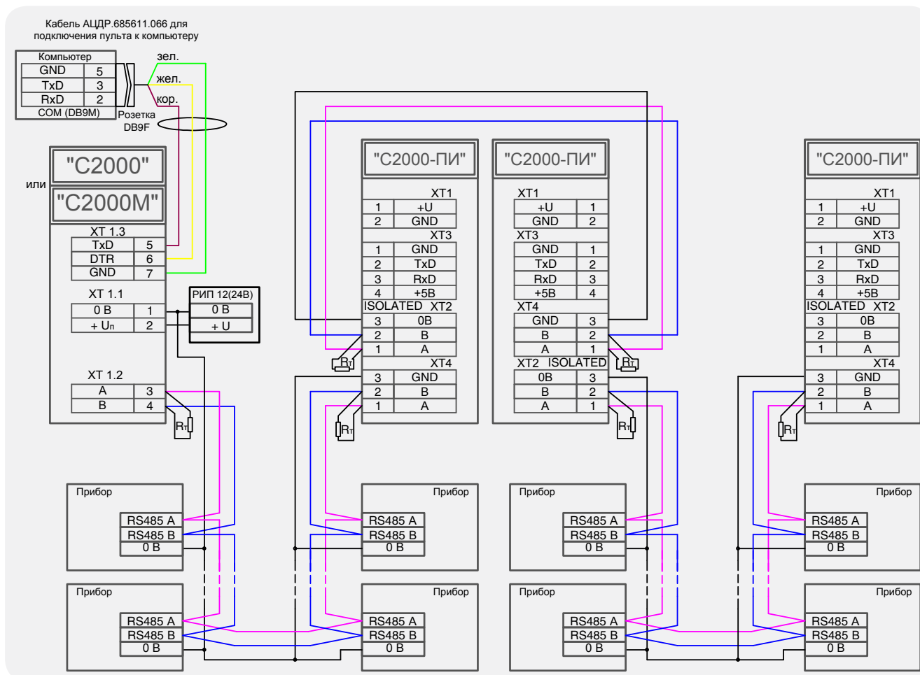
Рисунок 96. Увеличение длины линии RS-485 с помощью повторителей интерфейса
