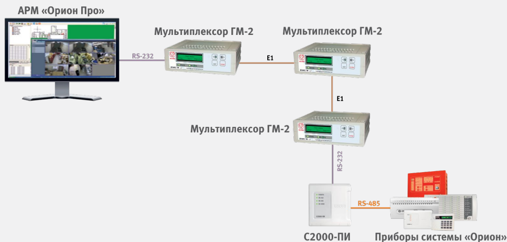
Рисунок 93. Структурная схема использования мультиплексора «ГМ-2» с АРМ «Орион»/«Орион Про» с подключением промежуточного мультиплексора (ремultipлексирование)
