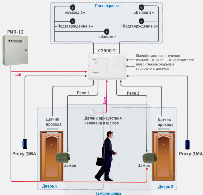
Рисунок 45. Режим работы «Шлюз»
