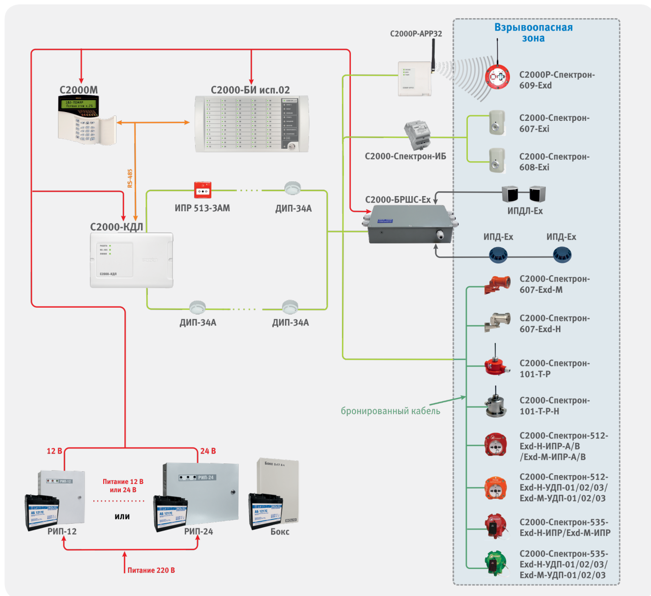
Рисунок 8. Взрывозащищенная система на базе адресно-аналоговой ПС
