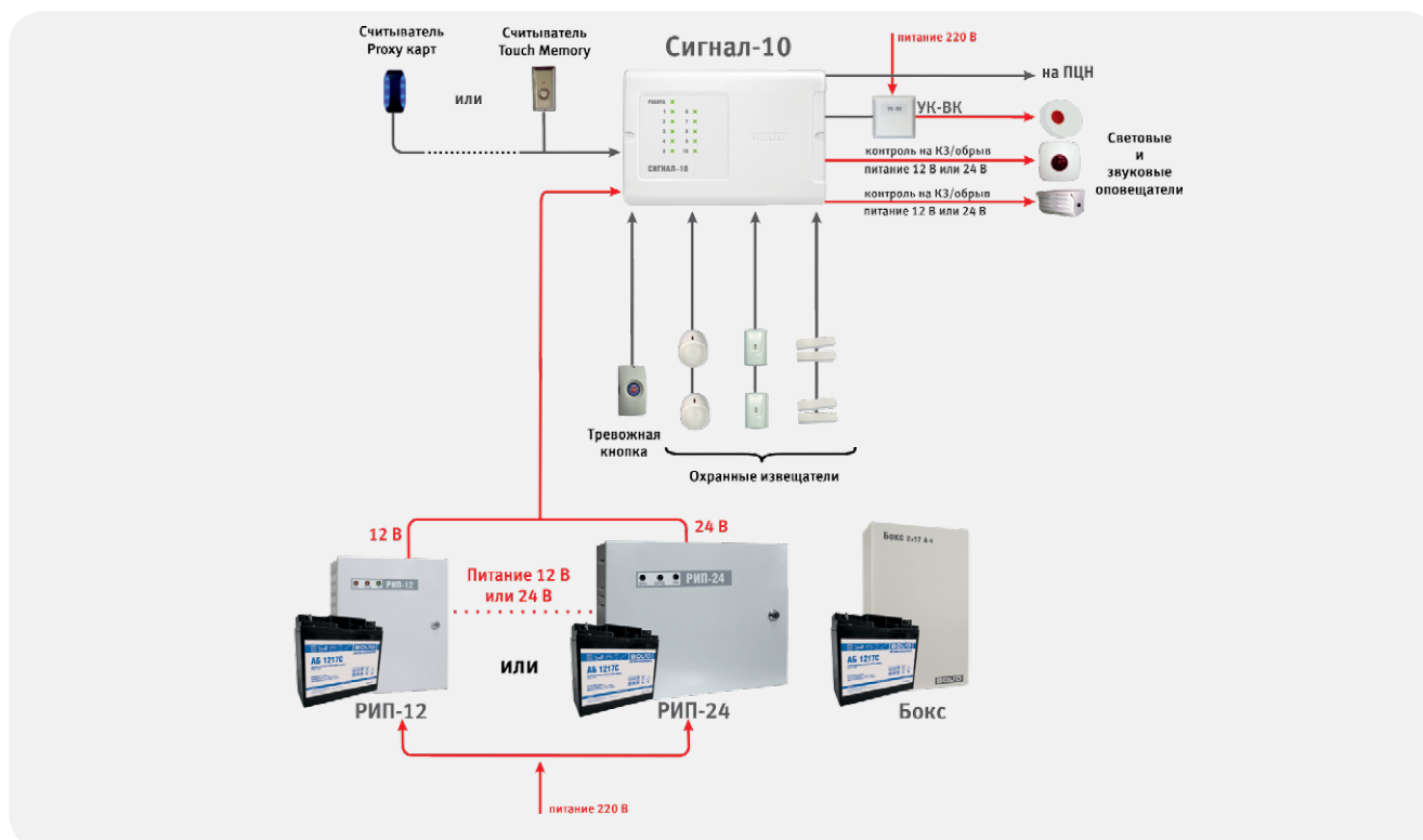
Рисунок 31. Автономное использование прибора «Сигнал-10»
