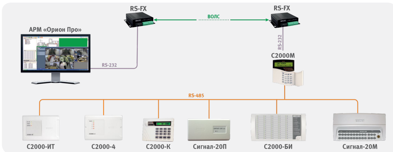
Рисунок 91. Типовая схема работы преобразователей RS-FX по протоколу «Орион Про»
