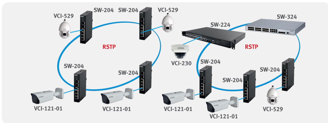
Рисунок 65. Примеры кольцевых топологий для построения периметральных систем видеонаблюдения
