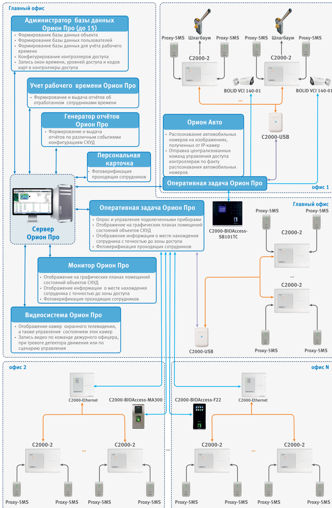
Рисунок 51. Системы контроля доступа с программным обеспечением
