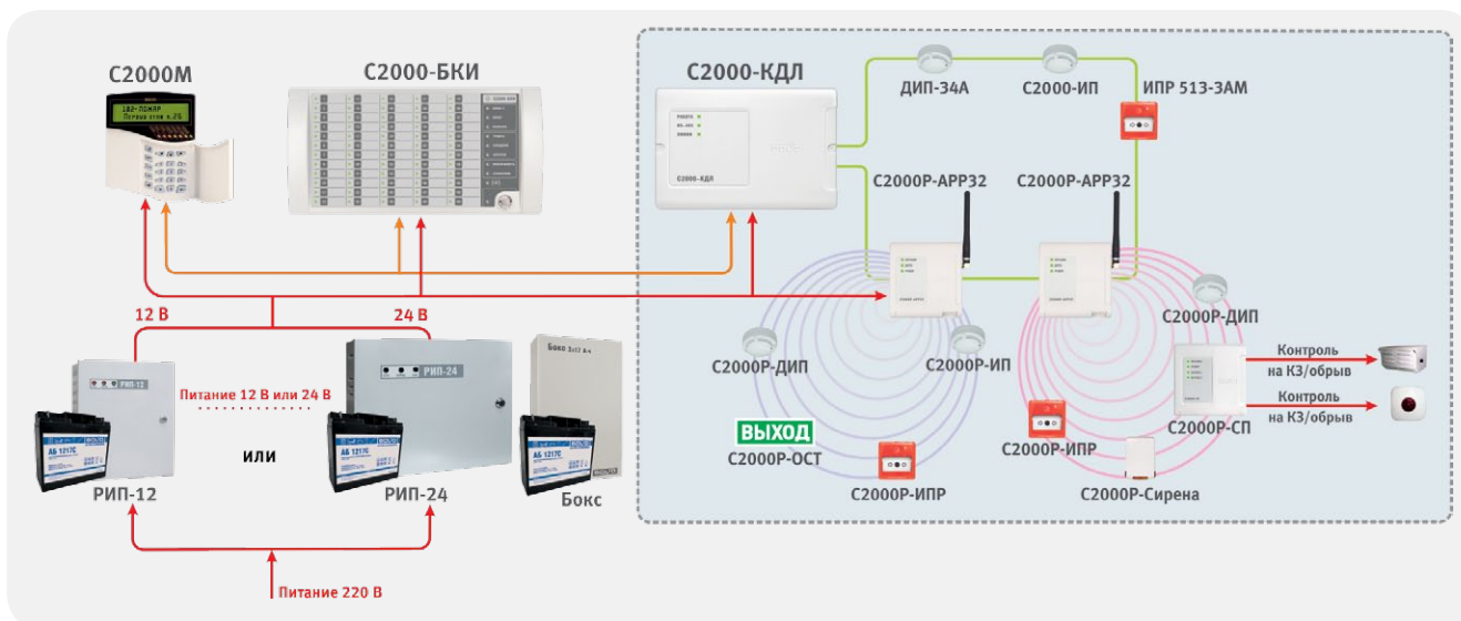
Рисунок 7. Радиоканальное расширение адресно-аналоговой системы пожарной сигнализации
