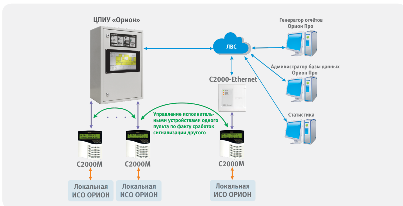
Рисунок 11. Организация перекрестных связей между пультами С2000М средствами ЦПИУ Орион
