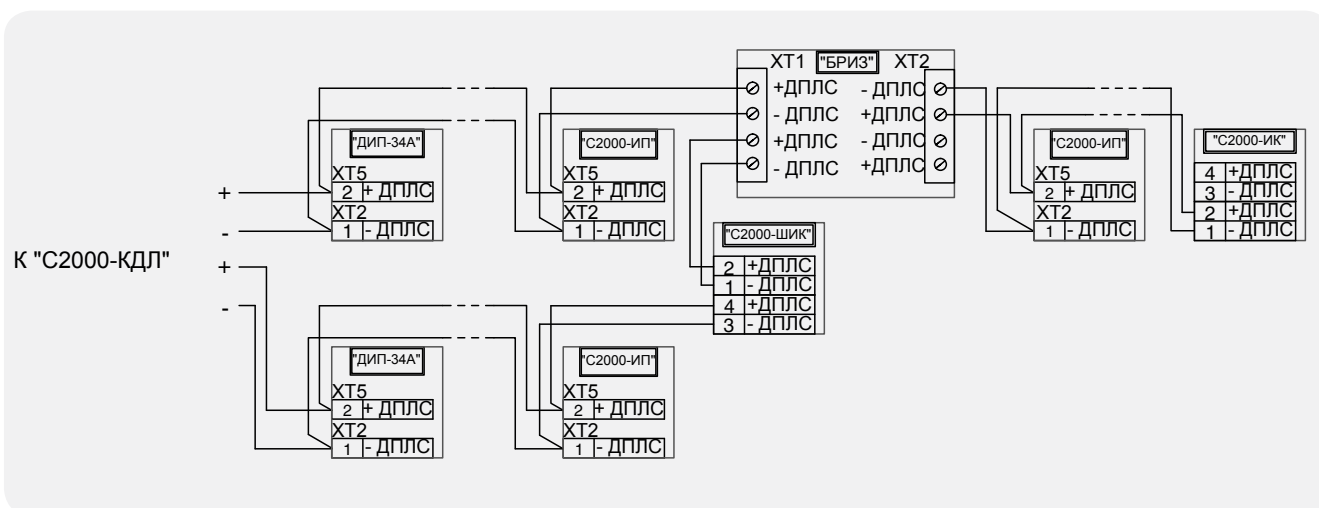
Рисунок 110. Схема подключения адресных извещателей в ДПЛС с топологией построения «кольцо»
