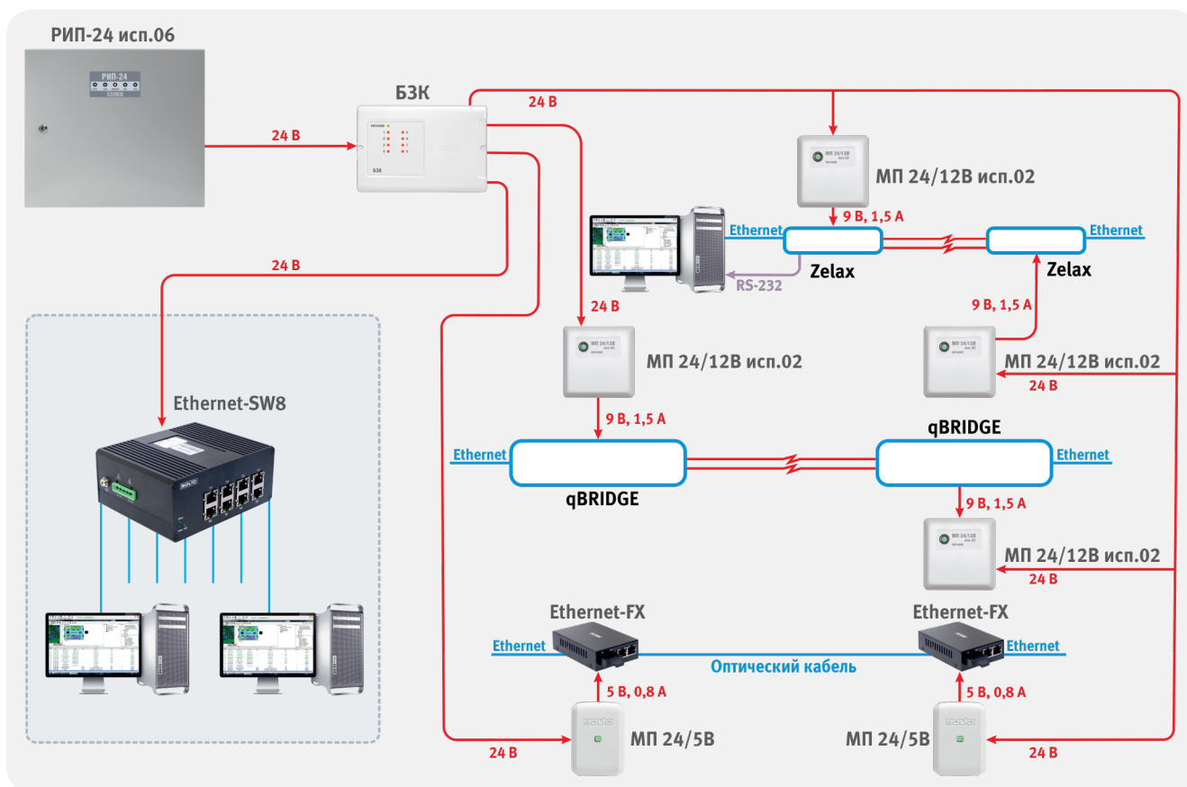
Рисунок 53. Электропитание сетевого каналобразующего оборудования
