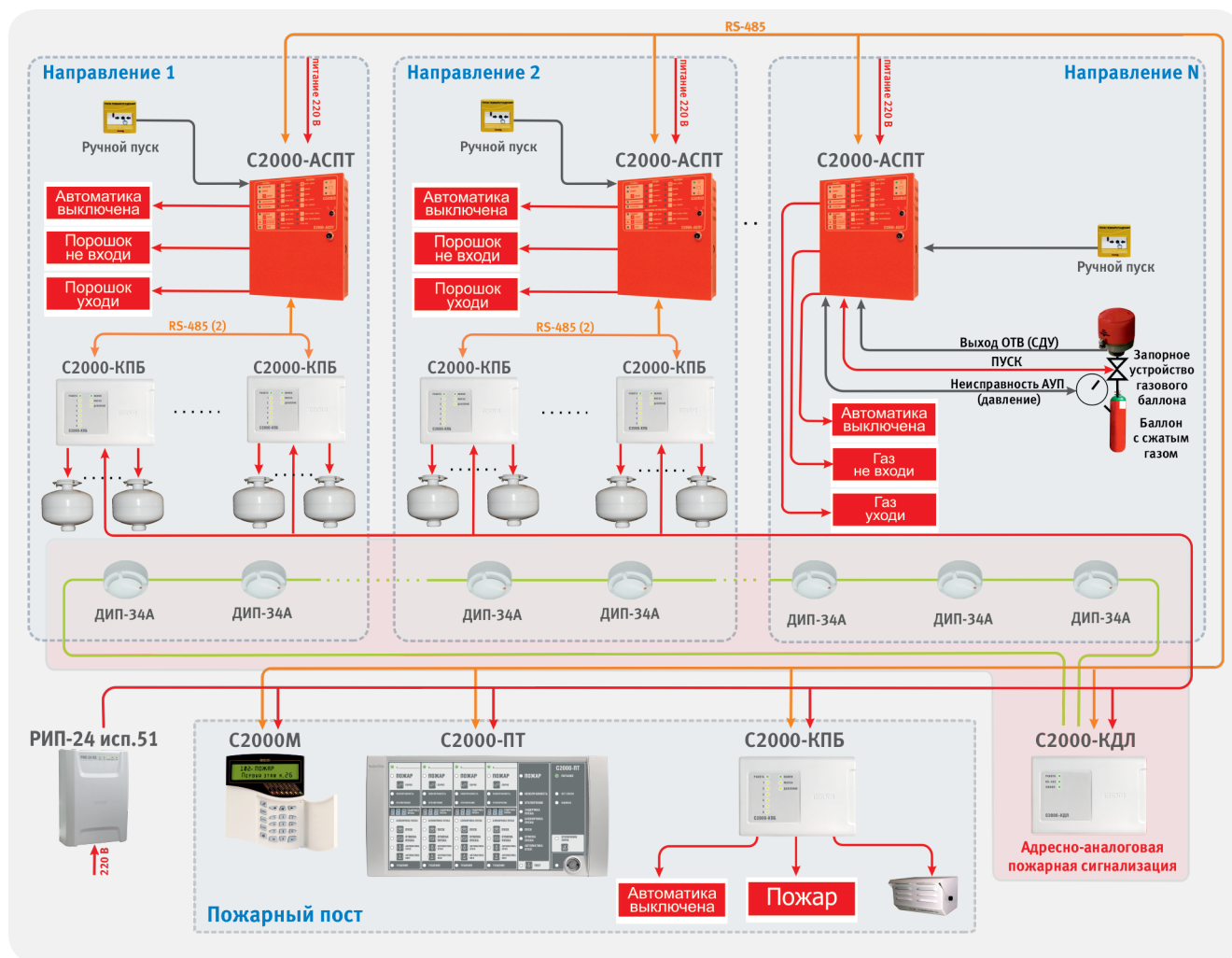
Рисунок 26. Система газового и порошкового тушения с использованием адресно-аналоговой пожарной сигнализации
