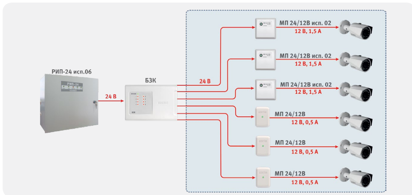
Рисунок 70. Организация электропитания системы видеонаблюдения
