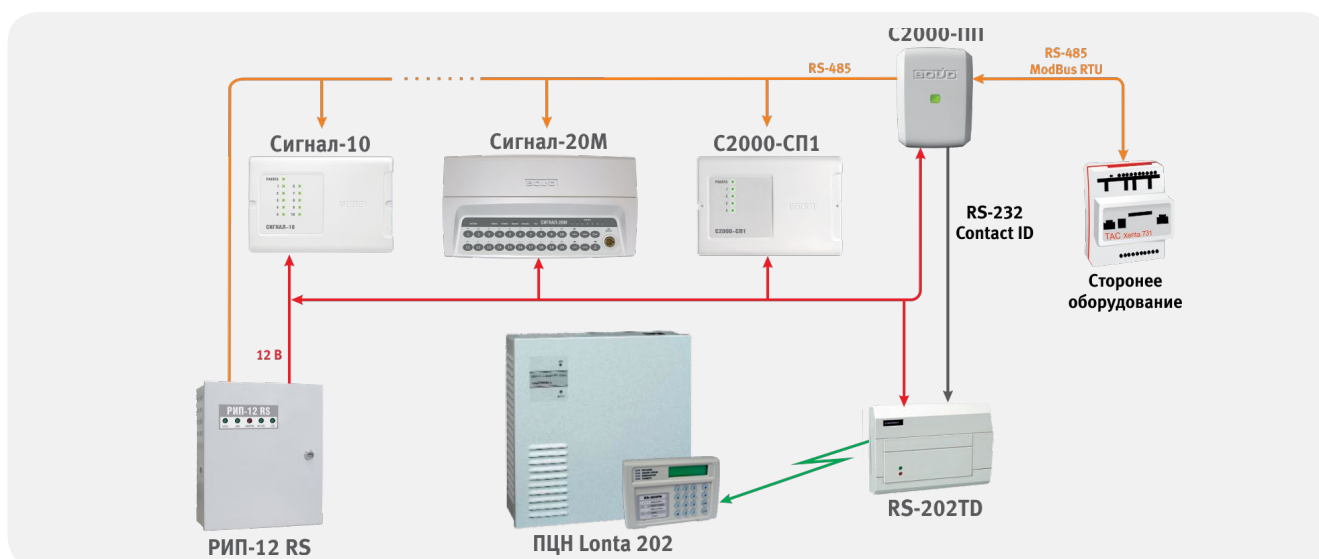
Рисунок 78. Применение «С2000-ПП» в ведущем режиме
