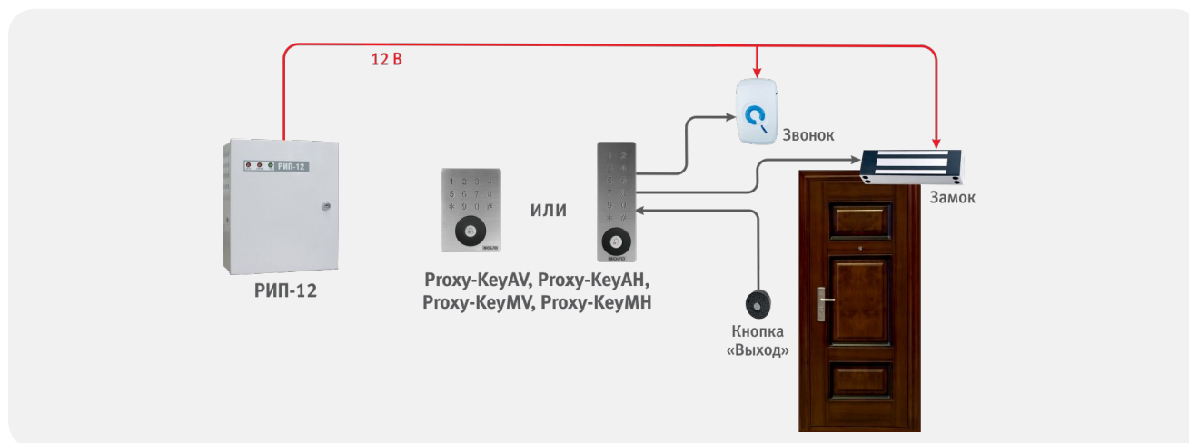
Рисунок 49. «Proxy-KeyAV/AH», «Proxy-KeyMV/MH»
