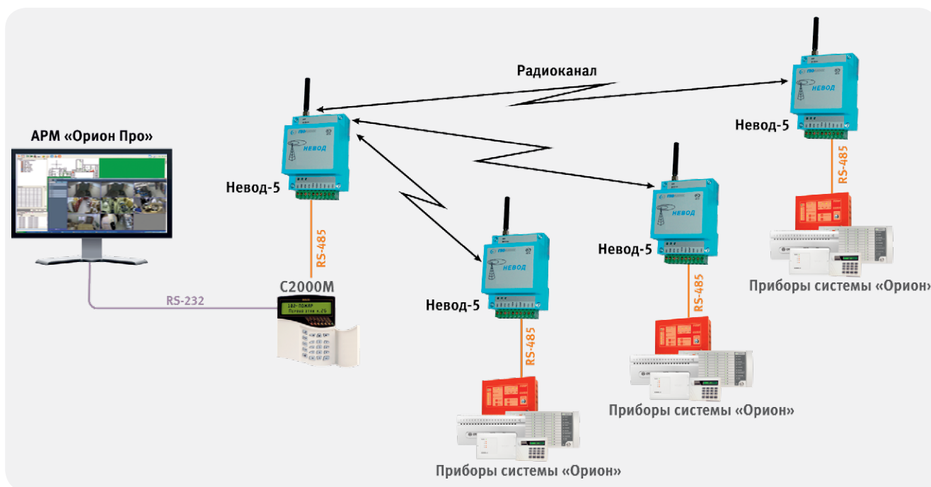
Рисунок 104. Структурная схема использования «Невод-5» с АРМ «Орион Про» и «С2000М», соединение «точка-многоточка»
