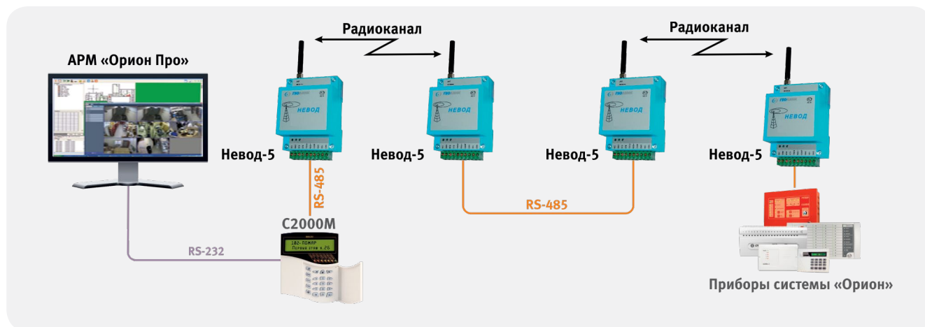
Рисунок 105. Структурная схема использования «Невод-5» с АРМ «Орион Про» и «С2000М», соединение «точка-точка» с ретрансляцией
