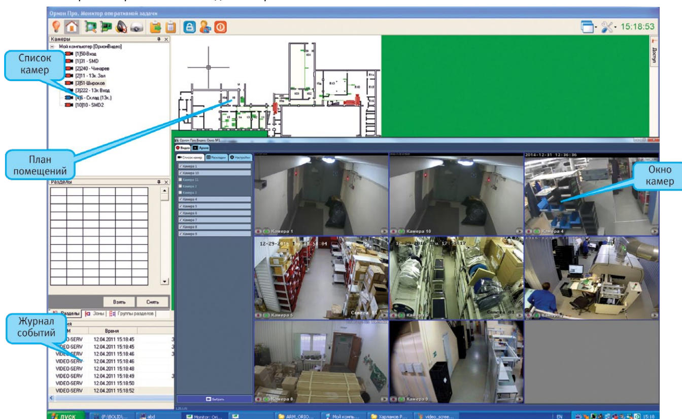
Рисунок 61. Пример рабочего интерфейса АРМ Орион Про
